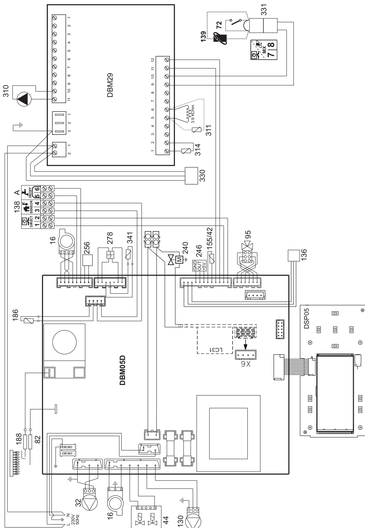
fig. 75 - Schema elettrico di serie
