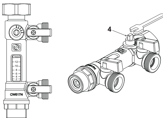
fig. 65 - Limitatore di portata
