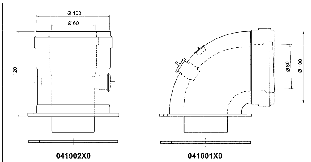
fig. 54 - Accessori di partenza per condotti coassiali
