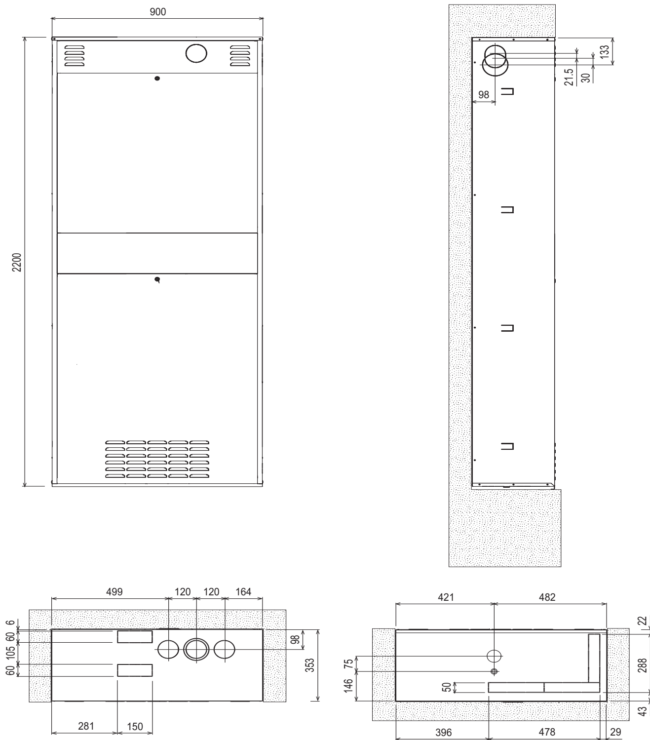
fig. 69 - Dimensioni involucro
