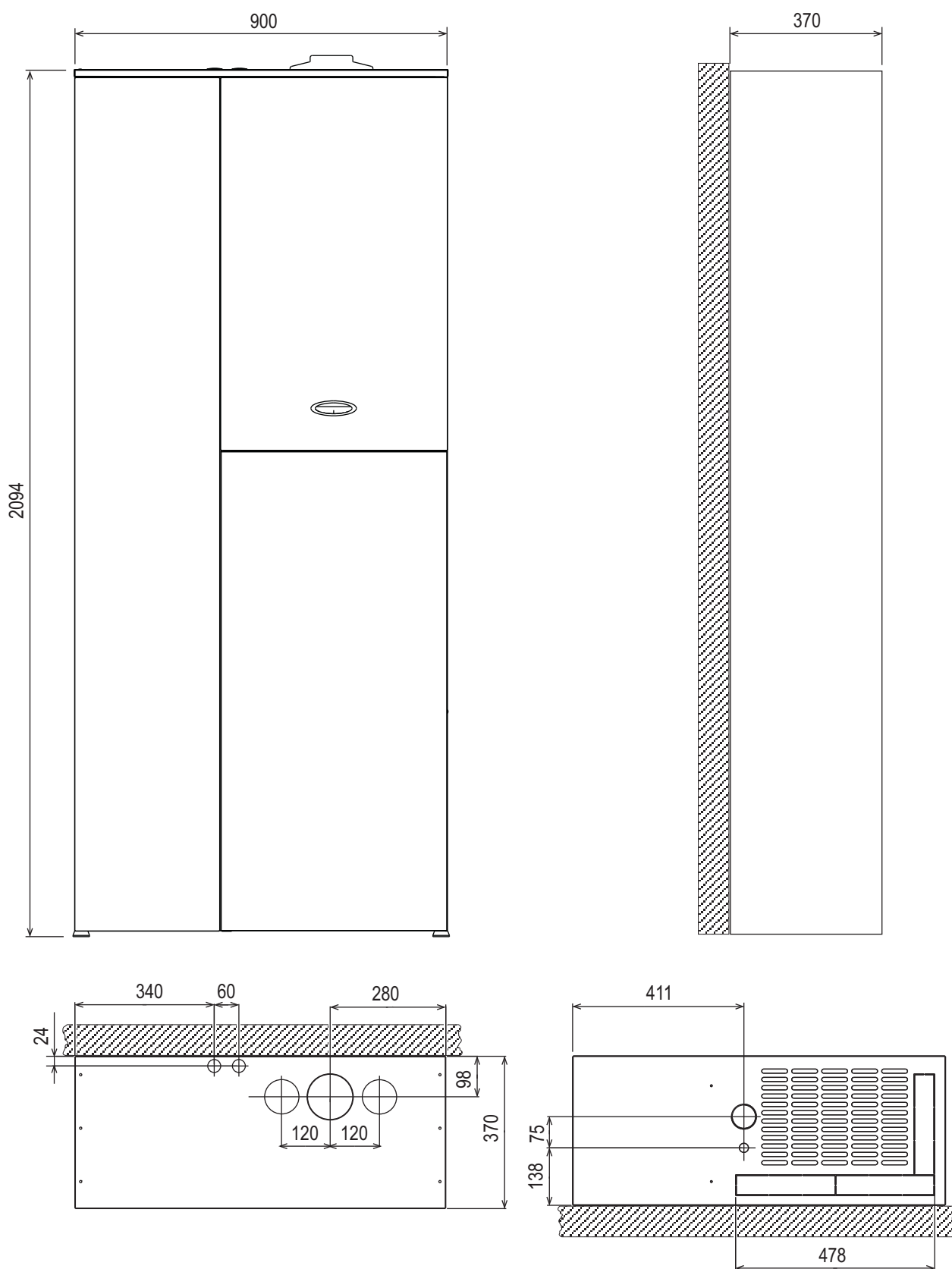
fig. 70 Dimensioni armadio
