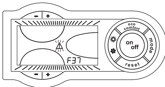
fig. 17 - Anomalia pressione impianto insufficiente
