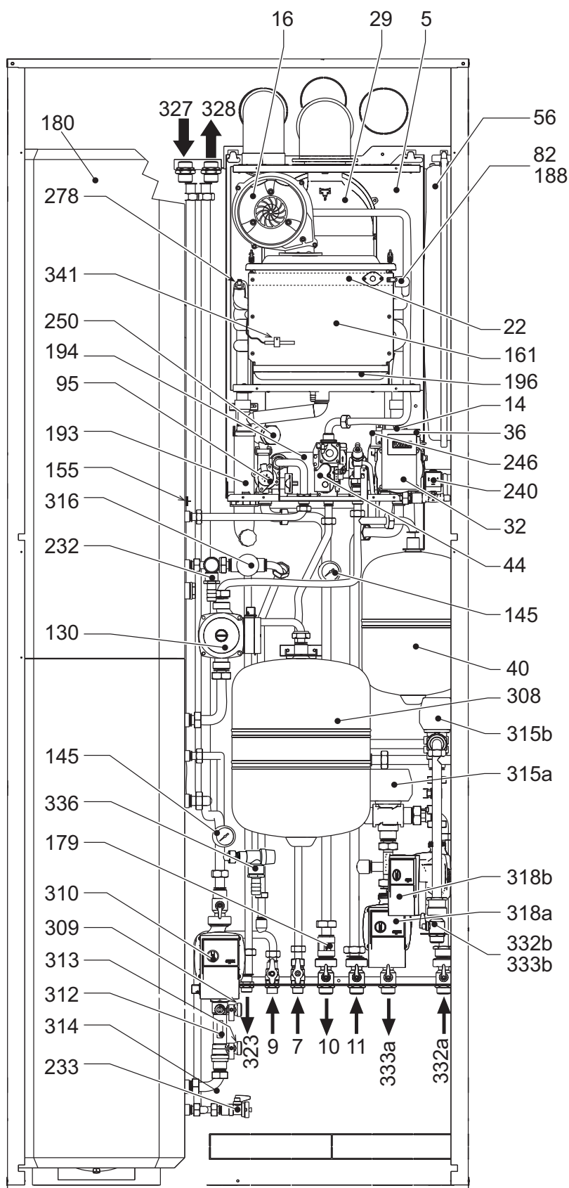
fig. 72 - Componenti principali versione COMPLETA
