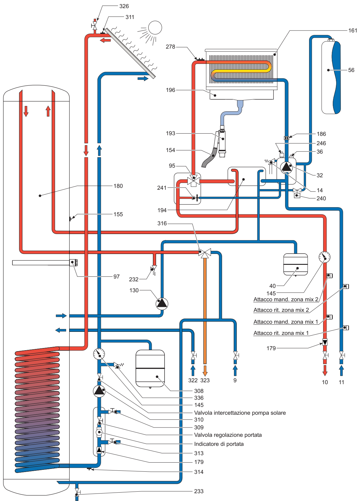
fig. 74 - Circuito idraulico configurazione COMPLETA
