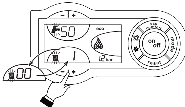
fig. 61 - Modalità TEST (potenza riscaldamento = 100%)
