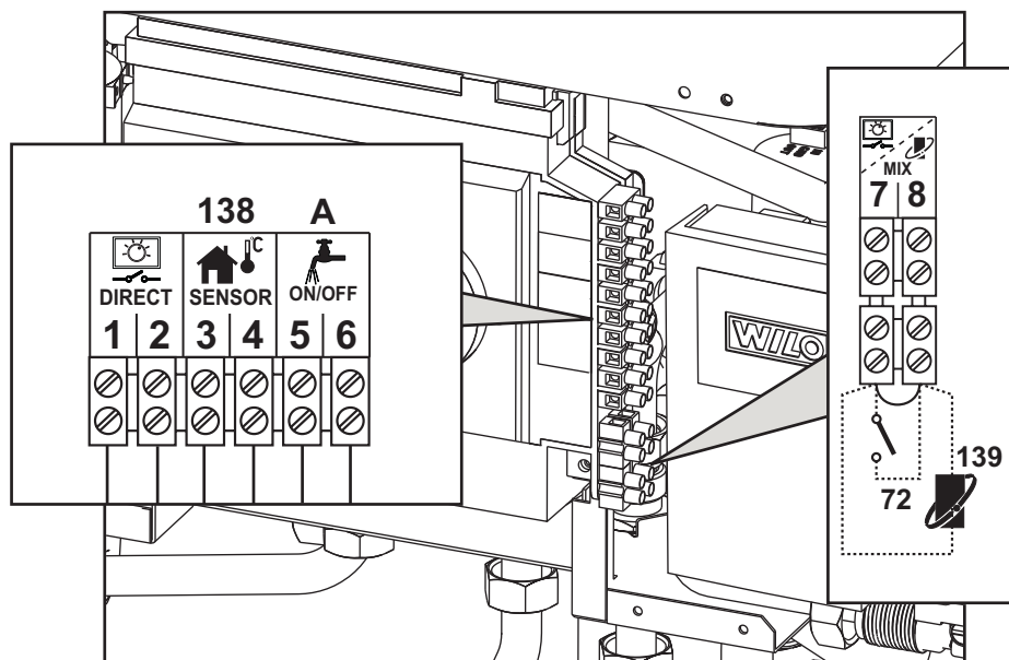
fig. 49 - Accesso alla morsettiera elettrica
