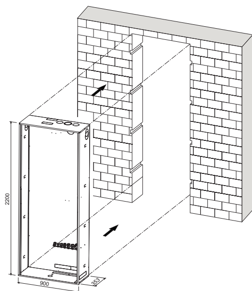
fig. 19 - Fissaggio dell'involucro ad incasso
