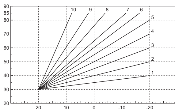
fig. 80 - Curve di compensazione
