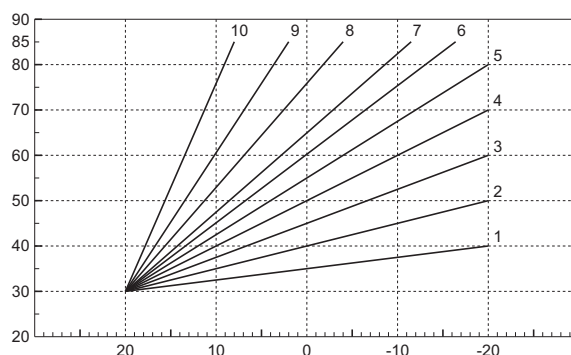
fig. 15 - Curve di compensazione
