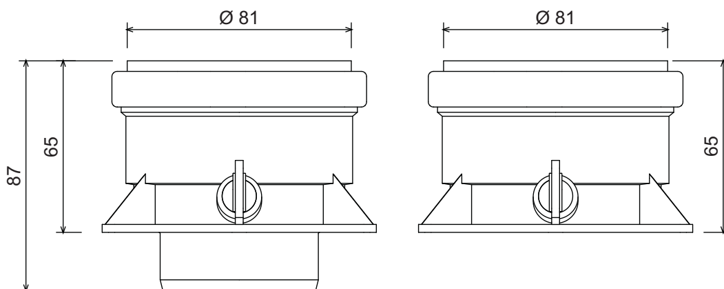
fig. 56 - Accessorio (cod. 041039X0) di partenza per condotti separati
