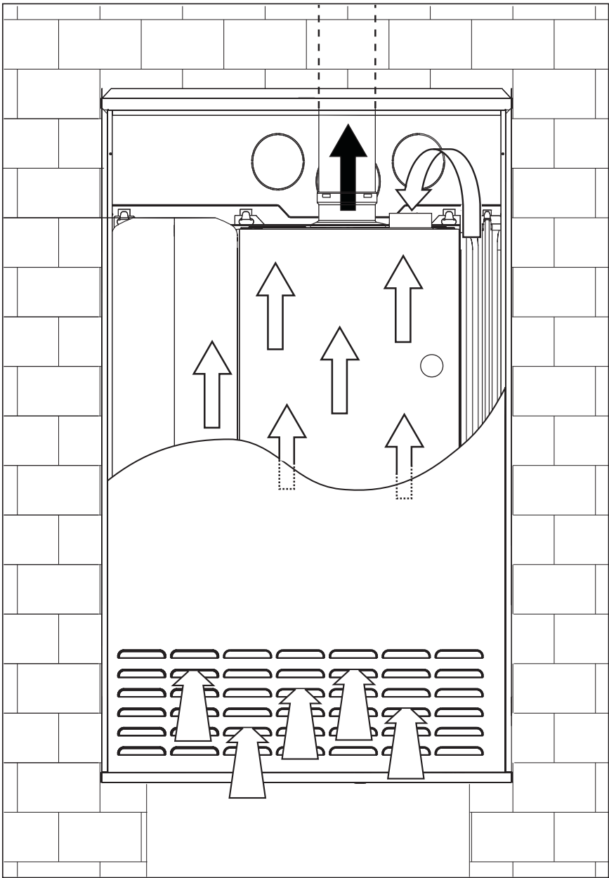
fig. 57 - Prelievo aria
