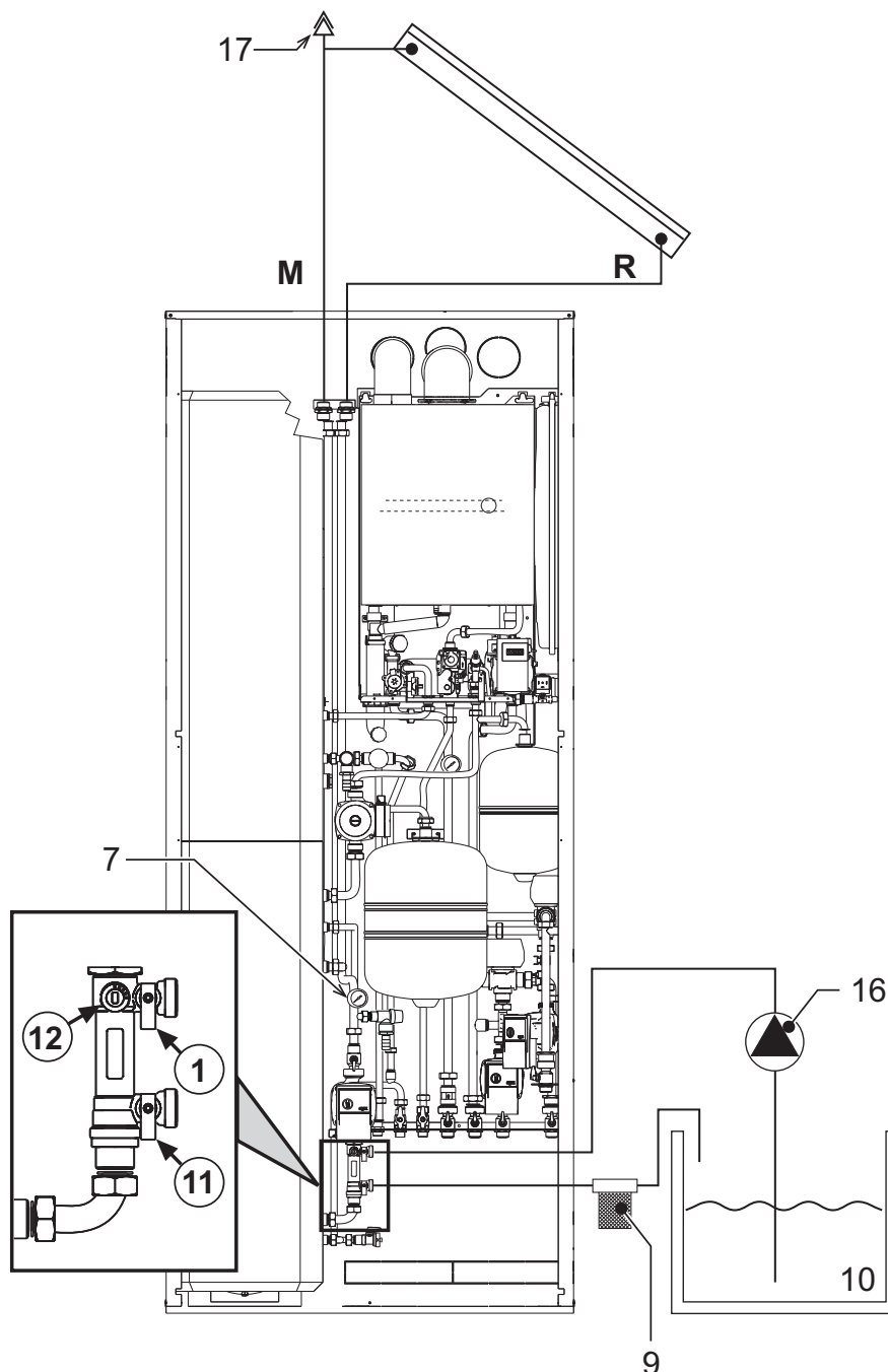
fig. 62 - Circuito solare
