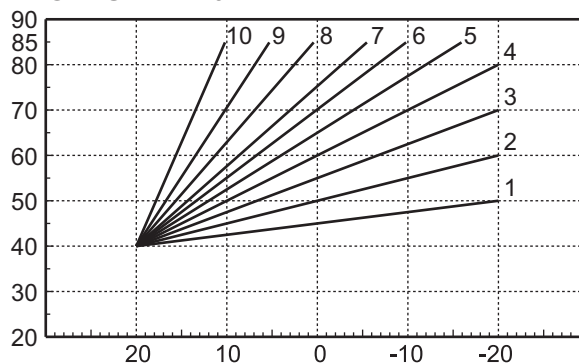
fig. 81 - Esempio di spostamento parallelo delle curve di compensazione
