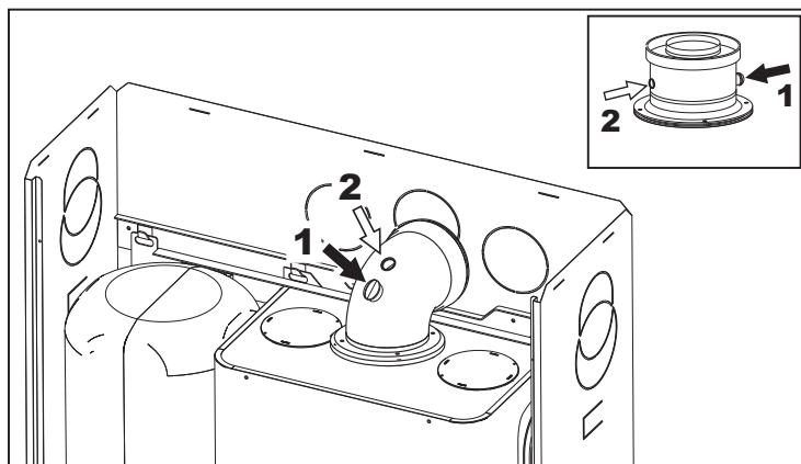
fig. 68 - Analisi della combustione
