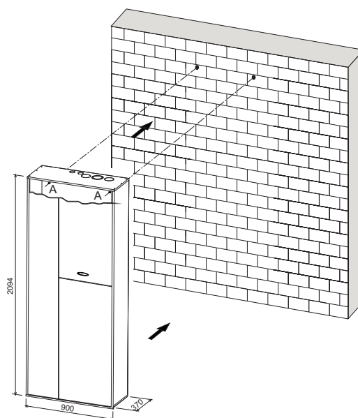
fig. 20 - Fissaggio dell'armadio a parete
