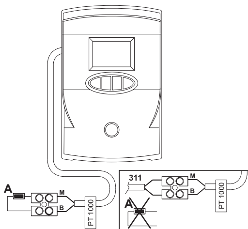
fig. 66 - Collegamento sensore collettore solare
