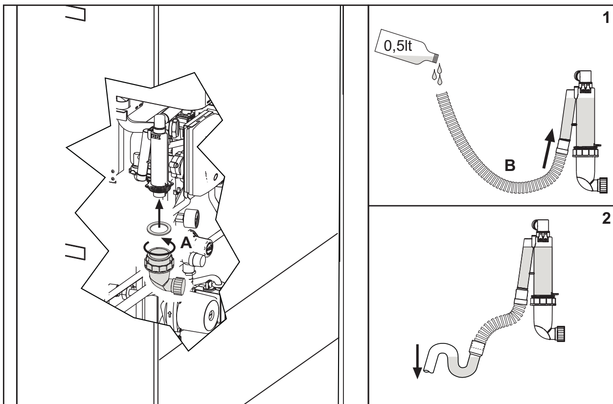
fig. 59 - Scarico condensa
