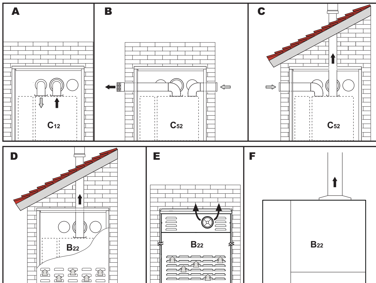
fig. 55 - Esempi di collegamento con tubi separati (⇨ = Aria / ⇨ = Fumi)
