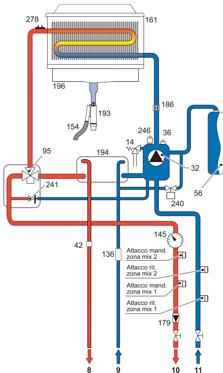
fig. 73 - Circuito idraulico configurazione BASE
