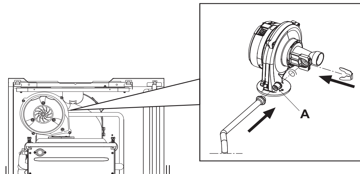
fig. 60 - Sostituzione ugello gas
