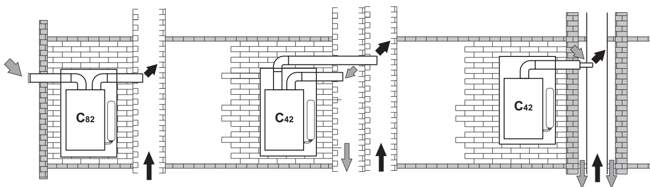
fig. 58 - Esempi di collegamento a canne fumarie (⇨ = Aria / ⇨ = Fumi)
