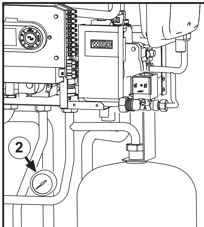
fig. 18 - Manometro interno
