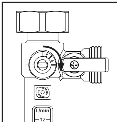
fig. 63 - Chiuso
