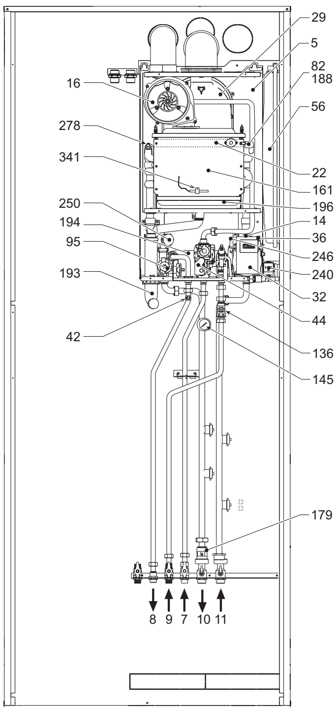
fig. 71 - Componenti principali versione BASE
