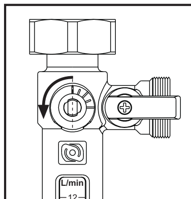
fig. 64 - Aperto
