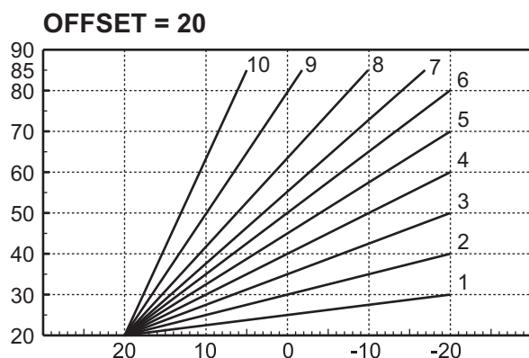
fig. 16 - Esempio di spostamento parallelo delle curve di compensazione
