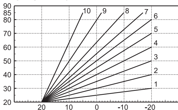
fig. 81 - Esempio di spostamento parallelo delle curve di compensazione
