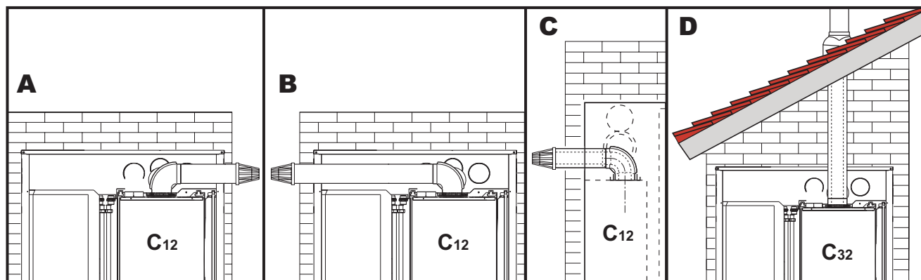
fig. 53 - Esempi di collegamento con tubi coassiali
