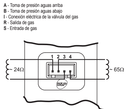
fig. 11 - Conexión de la válvula de gas
