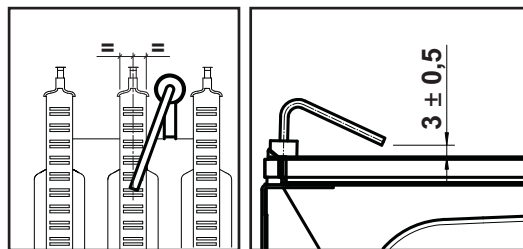
fig. 12 - Poziționarea electrodului
