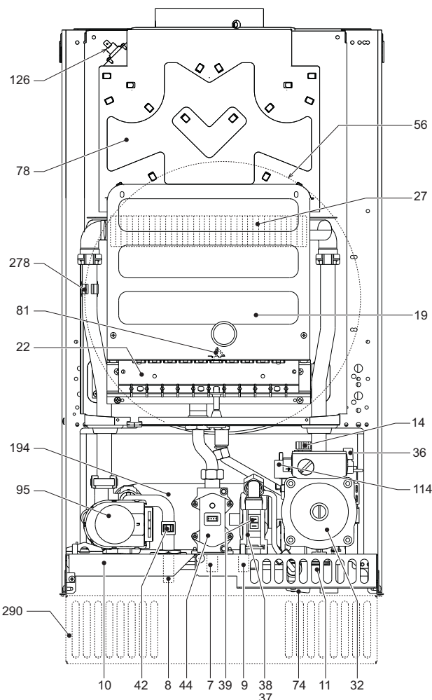
fig. 13 - Vue générale FL 24 MCA
