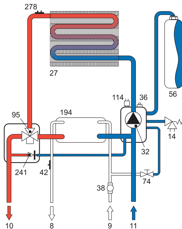
fig. 14 - Circuit Chauffage
