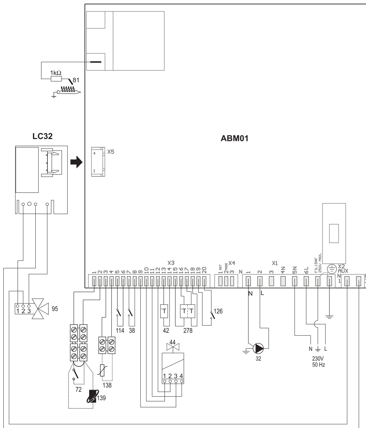
fig. 16 - Circuitul electric
