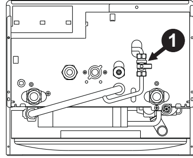
şek. 7 - Doldurma musluğu
