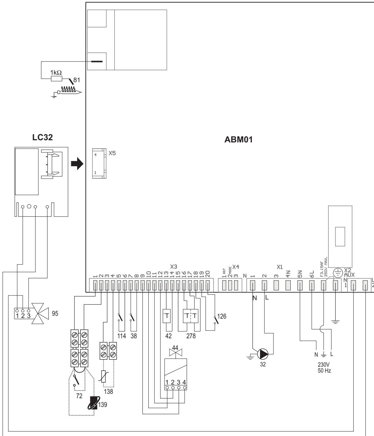
şek. 16 - Elektrik devresi
