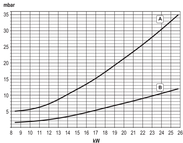
Pierderi de sarcină / înălțime de pompare pompe de circulație FL 24 MCA
