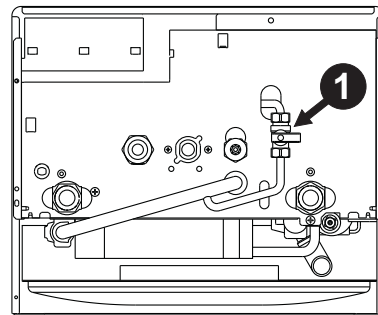
fig. 7 - Robinet de remplissage
