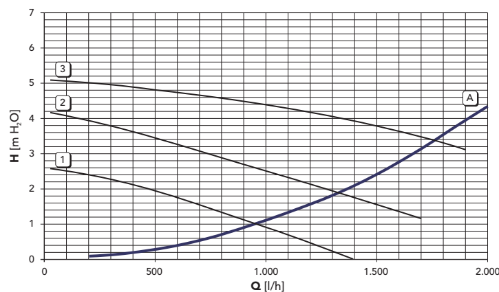
Pierderi de sarcină / înălțime de pompare pompe de circulație FL 24 MCA
