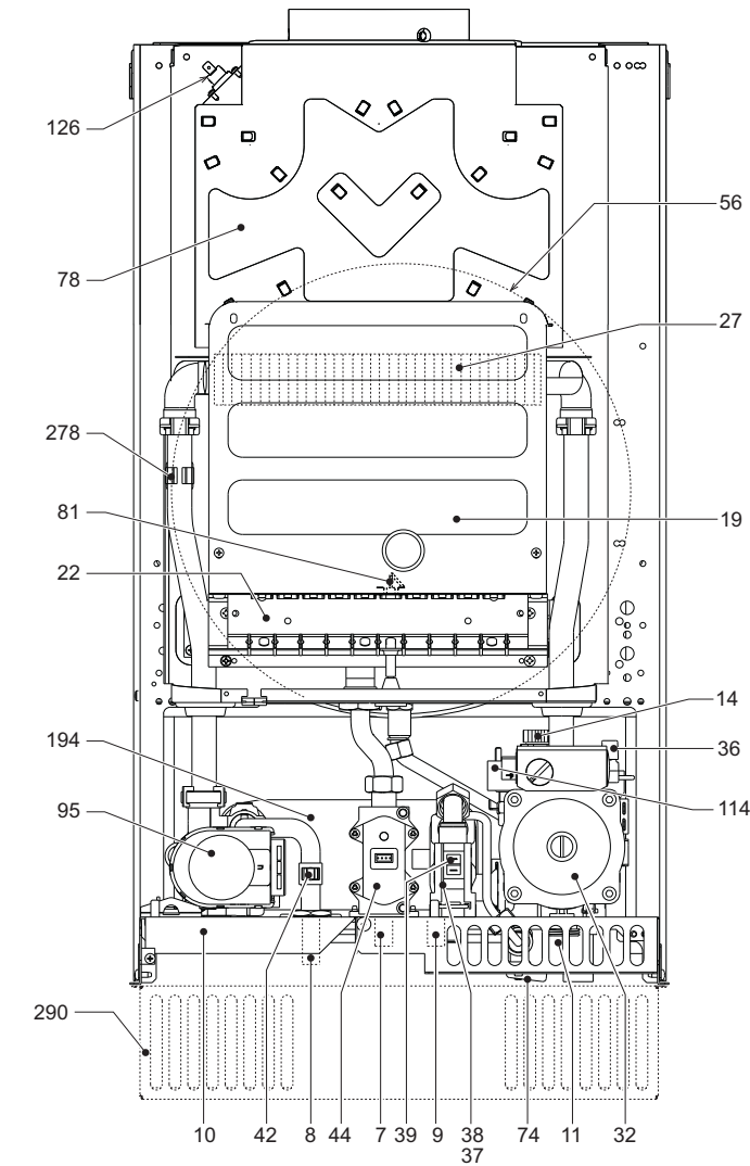
fig. 13 - Vista general FL 24 MCA
