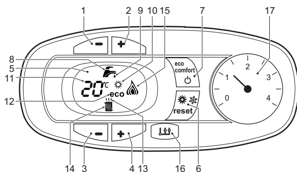
рис. 1 - Панель управления
