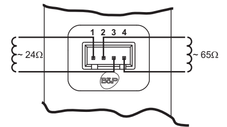
şek. 11 - Gaz valfi bağlantısı
