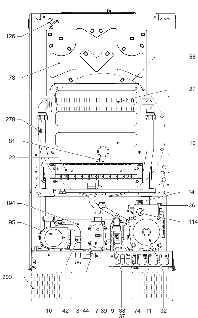
рис. 13 - Общий вид FL 24 MCA
