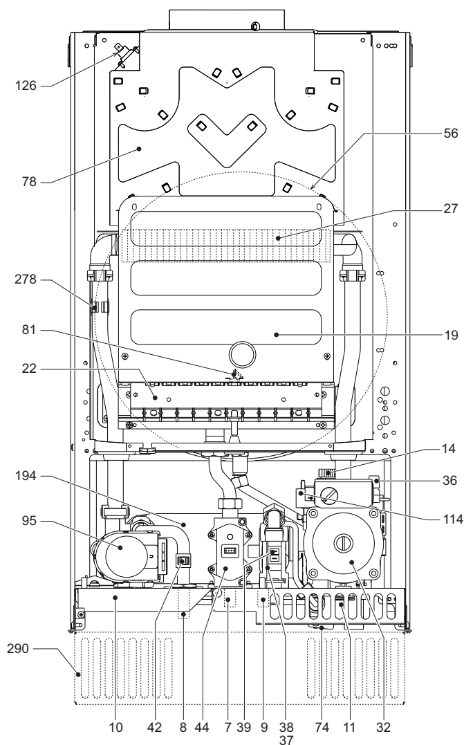
fig. 13 - Vedere generală FL 24 MCA
