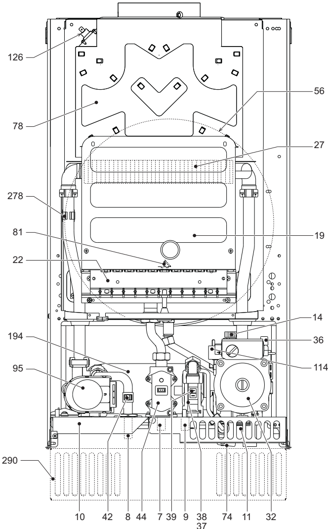
şek. 13 - Genel görünüm FL 24 MCA
