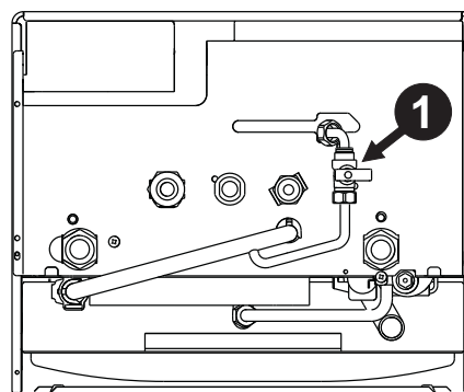
fig. 7 - Rubinetto di caricamento
