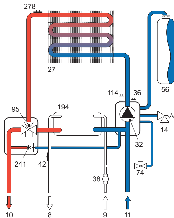
fig. 14 - Circuito riscaldamento
