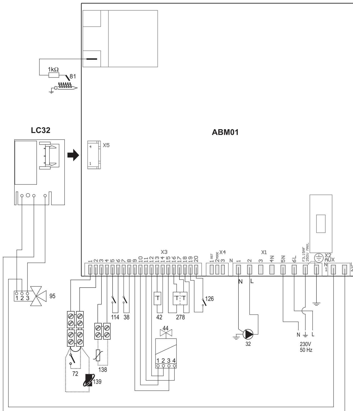
fig. 16 - Circuito elettrico
