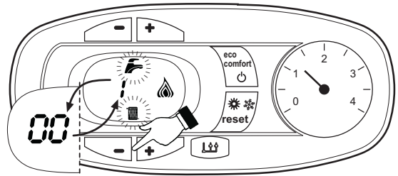
fig. 9 - Modalità TEST (potenza riscaldamento = 100%)
