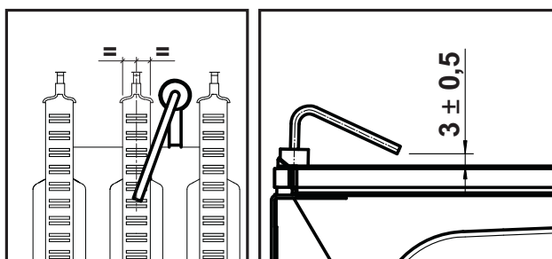
fig. 12 - Posizionamento elettrodo
