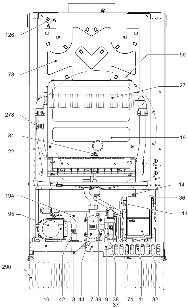
fig. 13 - Vista generale FL 24 MCA
