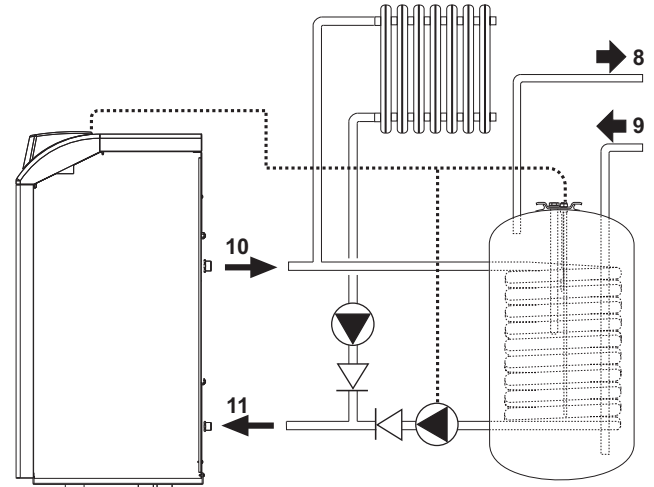
fig. 14 - Schema collegamento ad un bollitore esterno
