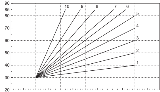
şek. 11 - Kompensasyon eğrisi
