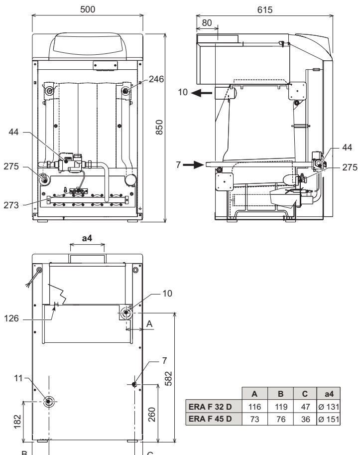
fig. 23 - Dimensioni e attacchi mod. ERA F 32 D e ERA F 45 D
