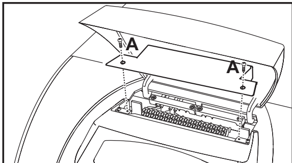
fig. 15 - Accesso alla morsetteria
