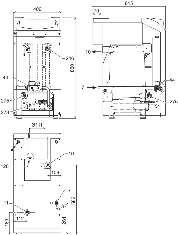
şek. 22 - Boyutlar ve eklentiler mod. ERA F 23 D
