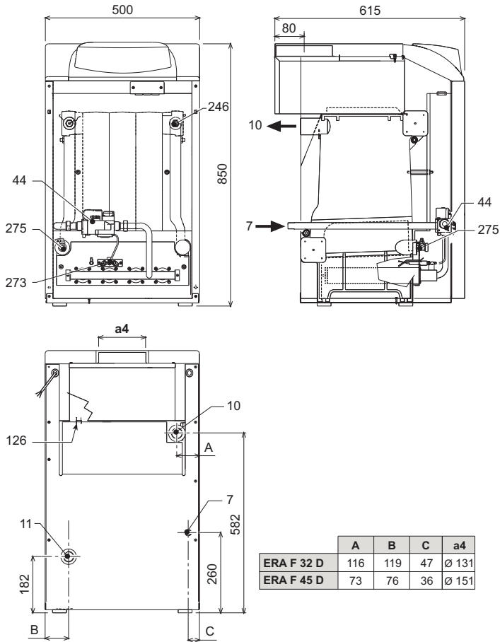
şek. 23 - Boyutlar ve eklentiler mod. ERA F 32 D e ERA F 45 D
