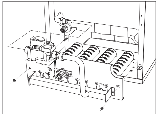
şek. 20 - Brülörlerin sökülmesi
