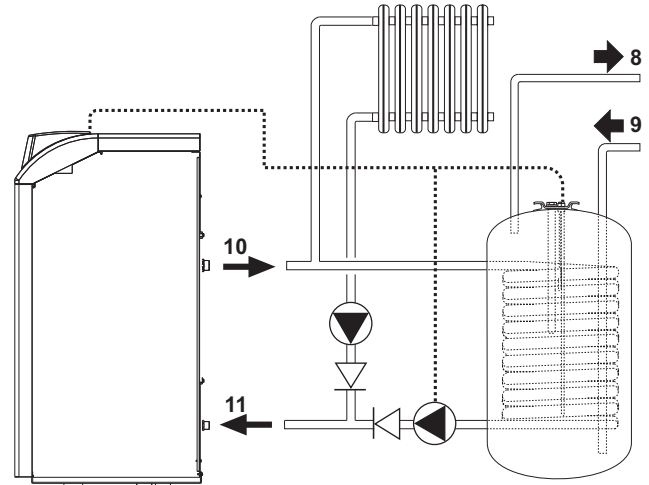
мал. 14 - Схема під'єднання до зовнішнього бойлера
