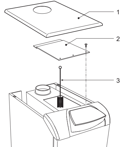
fig. 19 - Nettoyage de la chaudière
