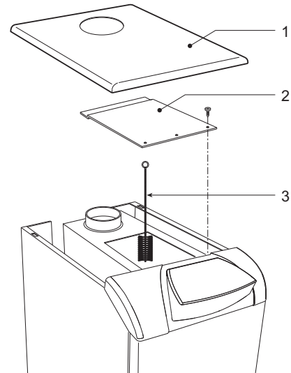
fig. 19 - Limpieza de la caldera
