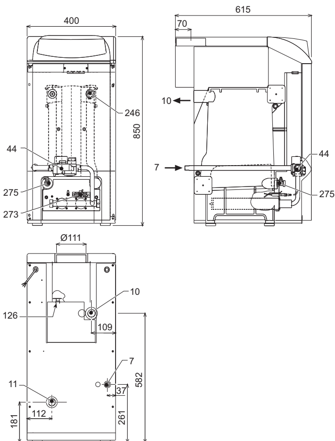
мал. 22 - Розміри і приєднувальні розміри мод. ERA F 23 D
