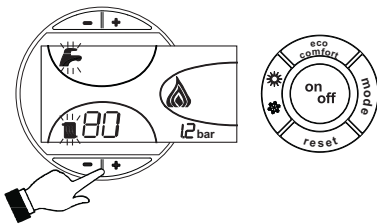
fig. 16 - Modo TEST
