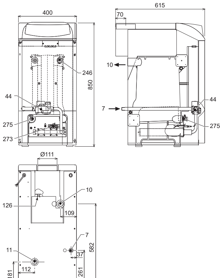
fig. 22 - Dimensioni e attacchi mod. ERA F 23 D
