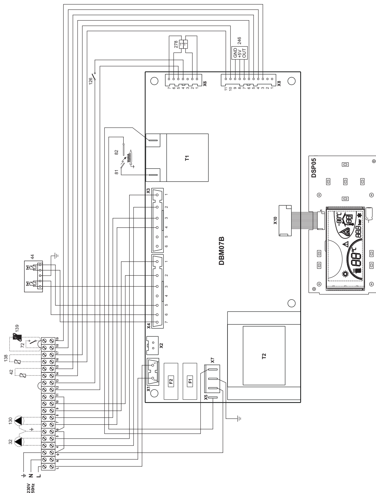
fig. 25 - Schéma électrique
