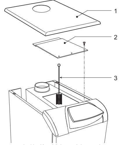
şek. 19 - Kombinin temizlenmesi
