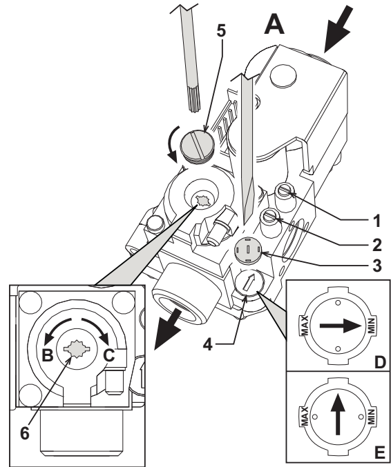
şek. 17 - Basıncın ayarlanması
