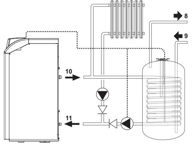
şek. 14 - Harici bir ısıtıcı kazanına bağlantı şeması
