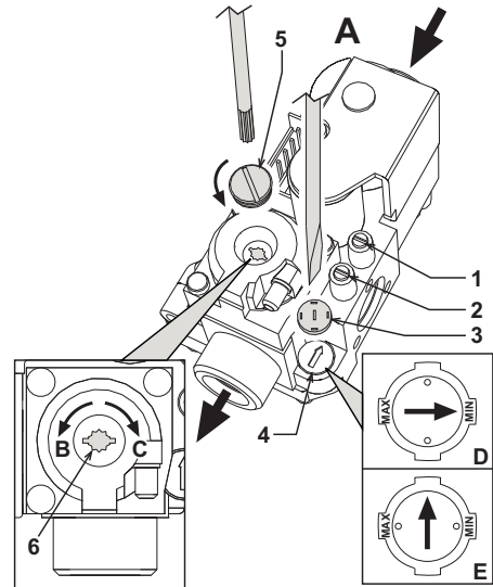
мал. 17 - Регулювання тиску
