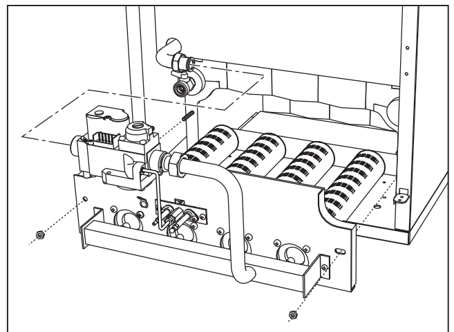
fig. 20 - Desmontaje de los quemadores
