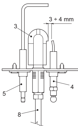
мал. 21 - Пілотний пальник
