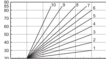
şek. 12 - Kompensasyon eğrilerinin paralel hareketine örnek
