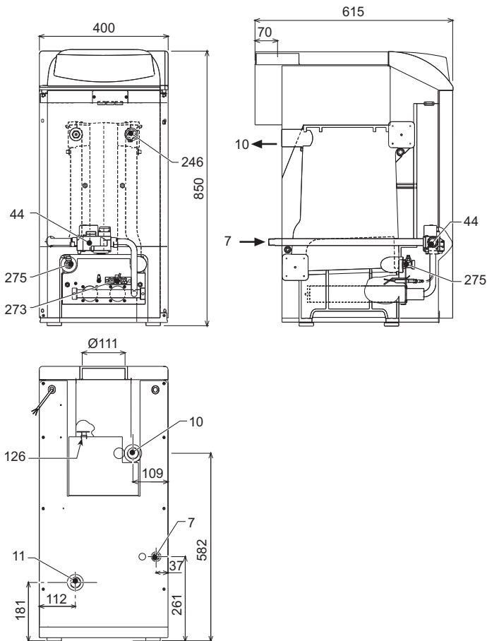
fig. 22 - Dimensions et raccords mod. ERA F 23 D
