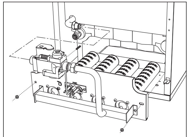
fig. 20 - Smontaggio bruciatori
