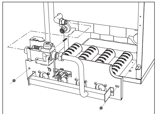
мал. 20 - Демонтаж пальників
