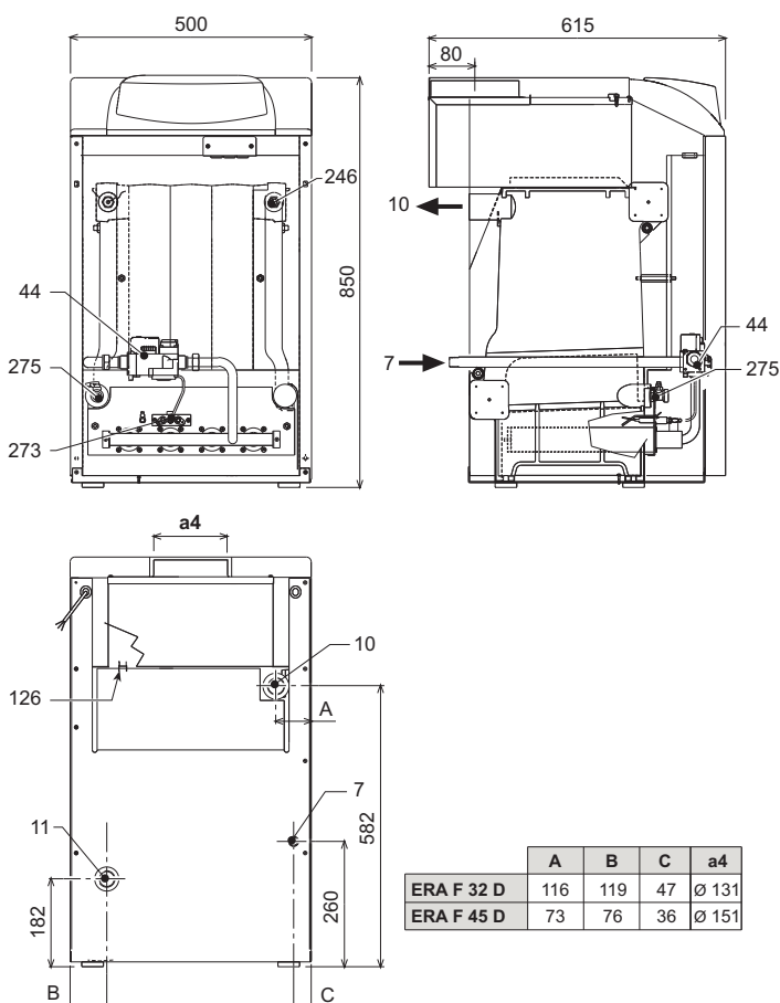
мал. 23 - Розміри, приєднання мод. ERA F 32 D E ERA F 45 D
