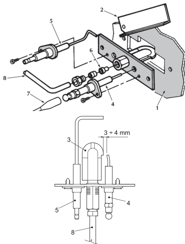
fig. 21 - Quemador piloto
