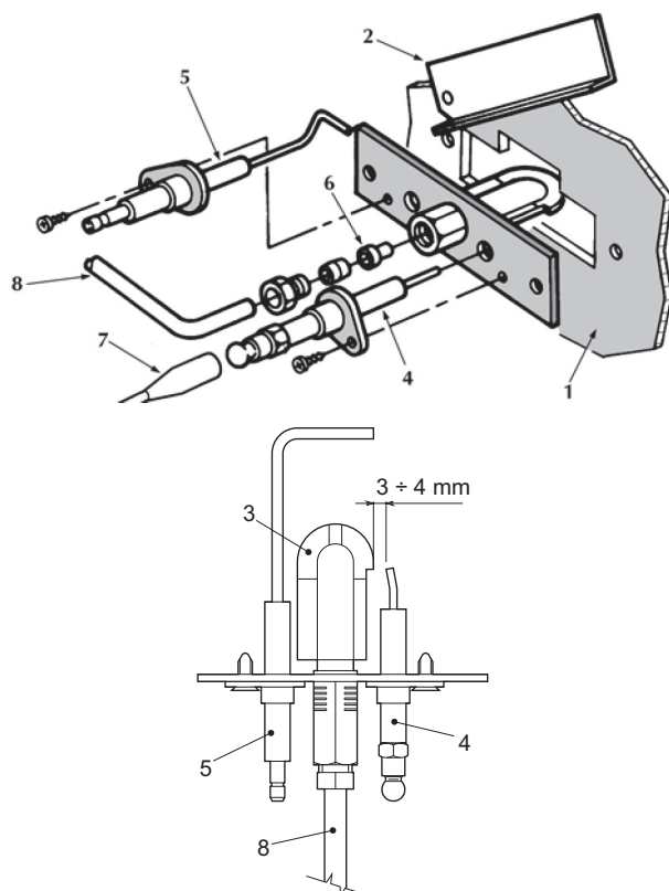
fig. 21 - Bruciatore pilota
