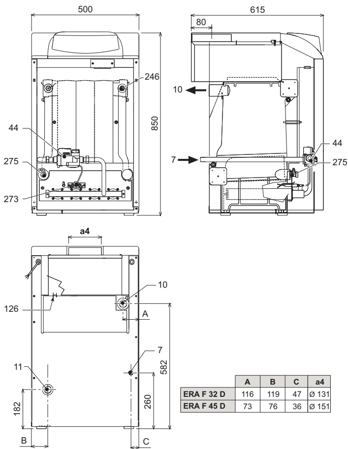
fig. 23 - Dimensions et raccords mod. ERA F 32 D E ERA F 45 D
