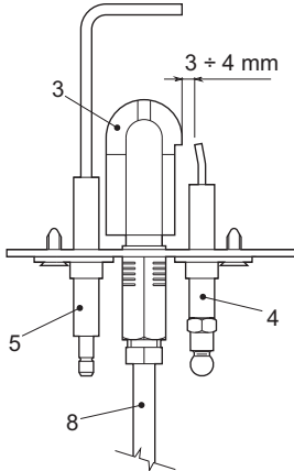
şek. 21 - Pilot brülör
