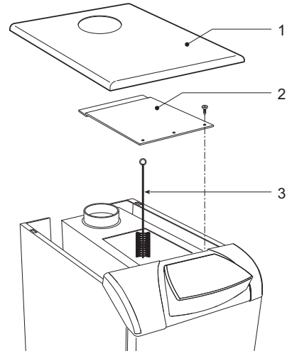
fig. 19 - Pulizia caldaia
