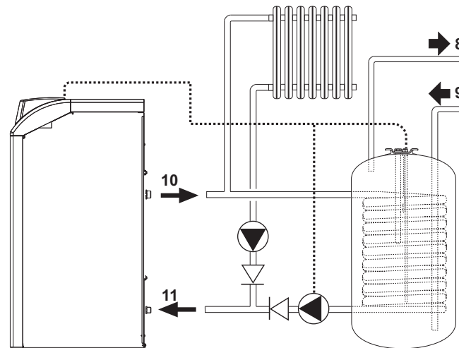
fig. 14 - Schéma de branchement à un ballon externe
