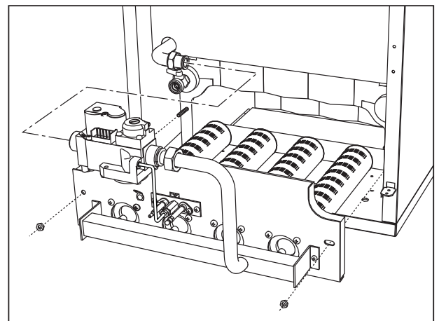
fig. 20 - Démontage des brûleurs
