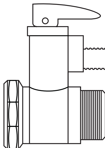
fig. 14 - Valvola di sicurezza 7 bar (0.7 MPa)
