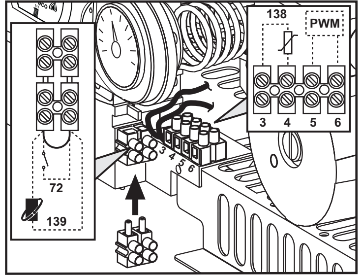
fig. 10 - Accès au bornier
