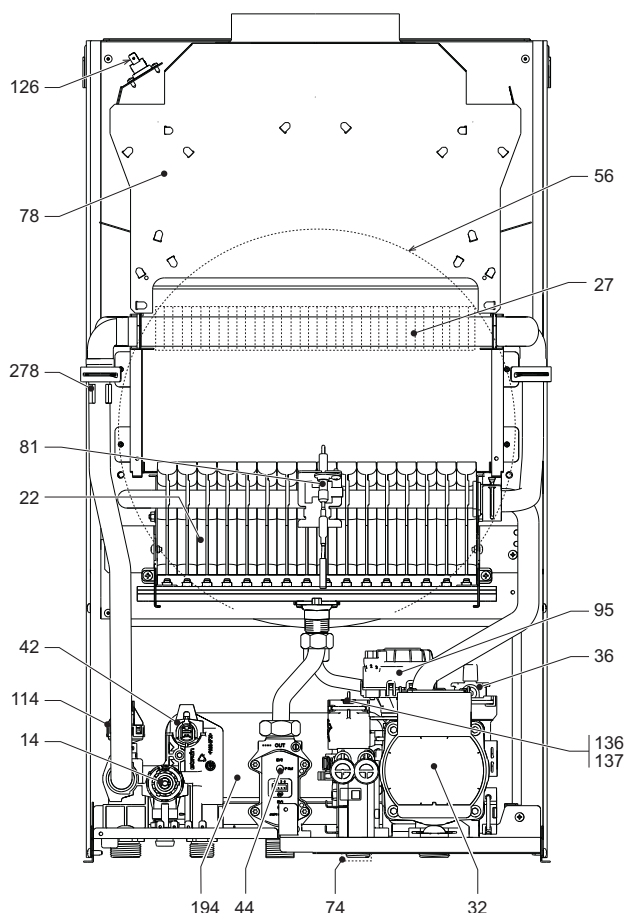
fig. 21- Vue générale - FL D LN C30
