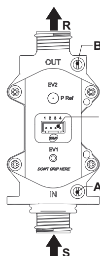
fig. 11 - Vanne à gaz
