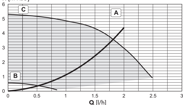
рис. 30 - Потеря напора/Напор циркуляционных насосов iXinox B 32 K 50
