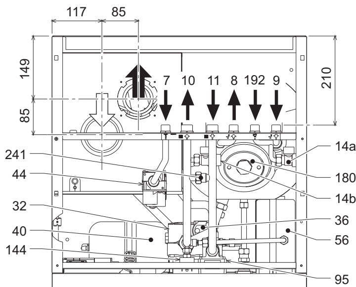
рис. 27 - Вид сзади
