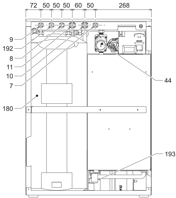
fig. 27 - Vista posteriore
