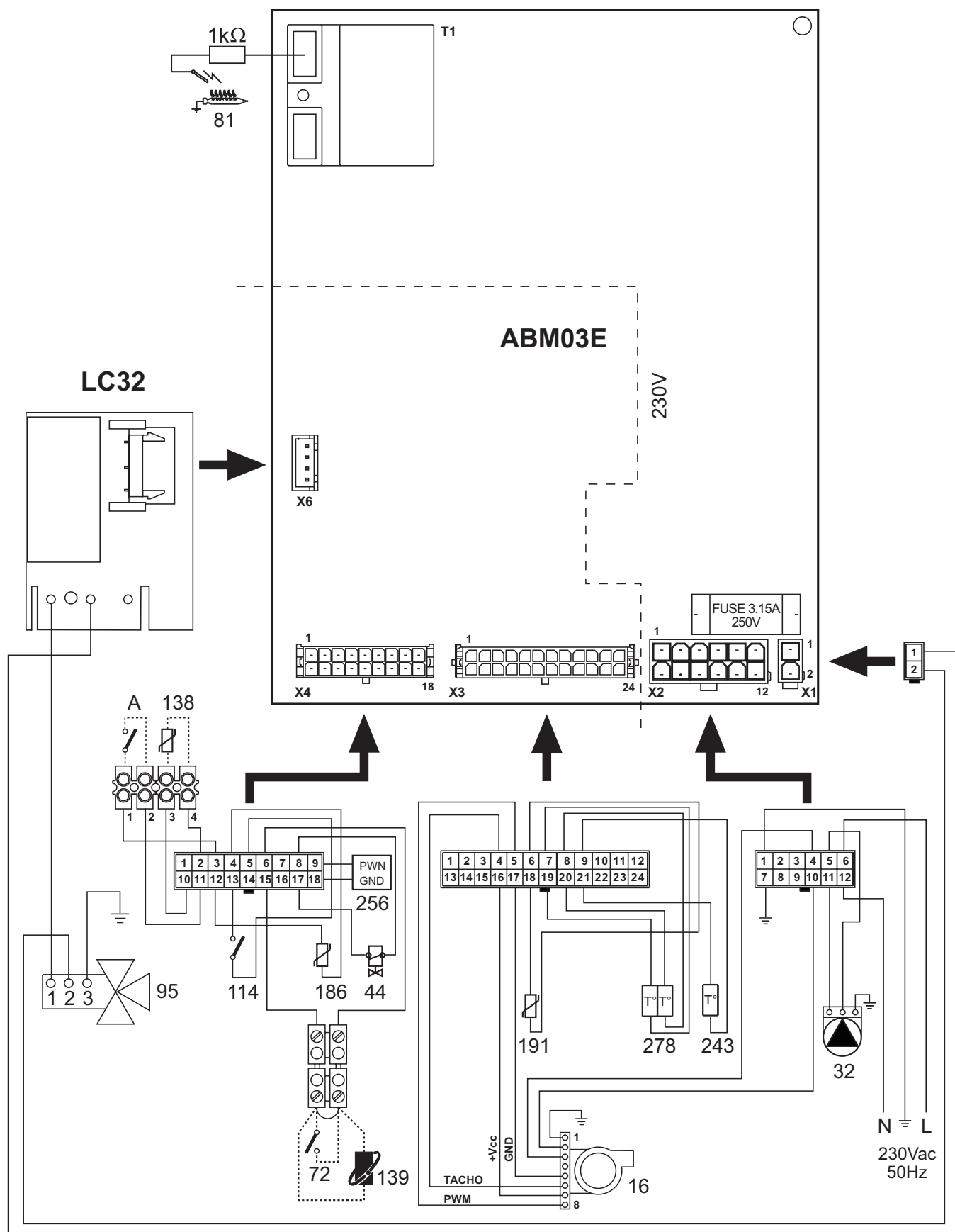
рис. 31 - Электрическая схема
