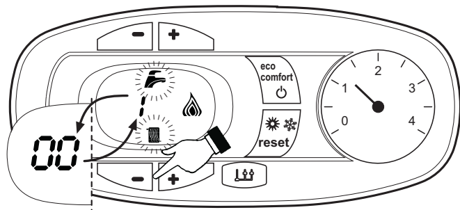
рис. 23 Режим TEST (мощность системы отопления = 100%)
