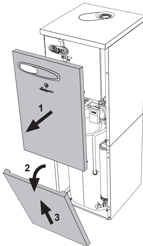
fig. 24 - Apertura pannello frontale
