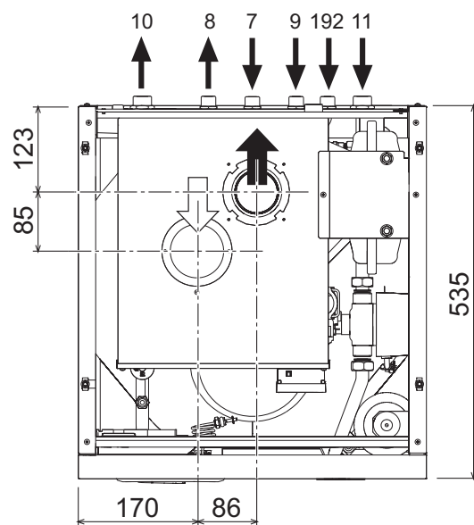
рис. 27 - Вид сверху (ВХОД ВОЗДУХА = / ОТВОД ДЫМА = )
