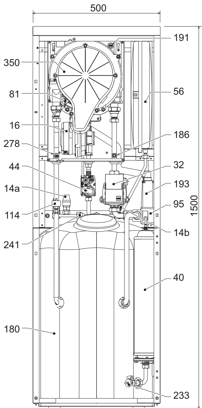
fig. 25 - Vista frontale
