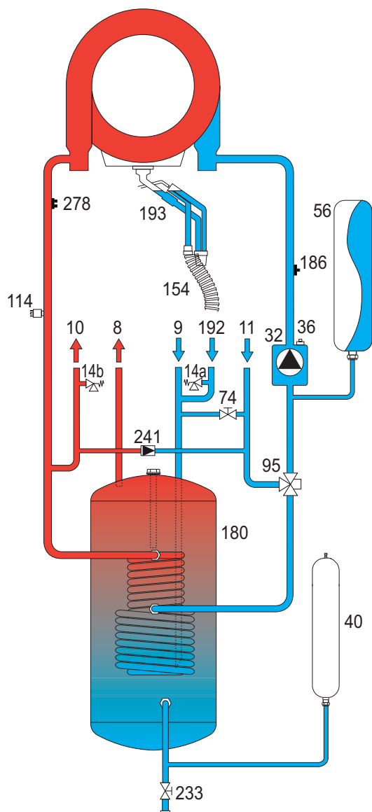
рис. 28 - Гидравлический контур
