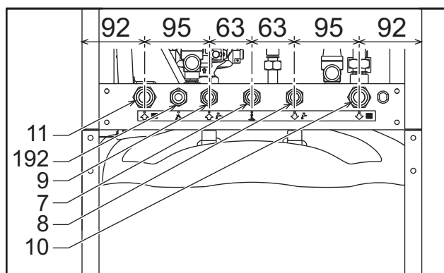
fig. 13 - Attacchi idraulici
