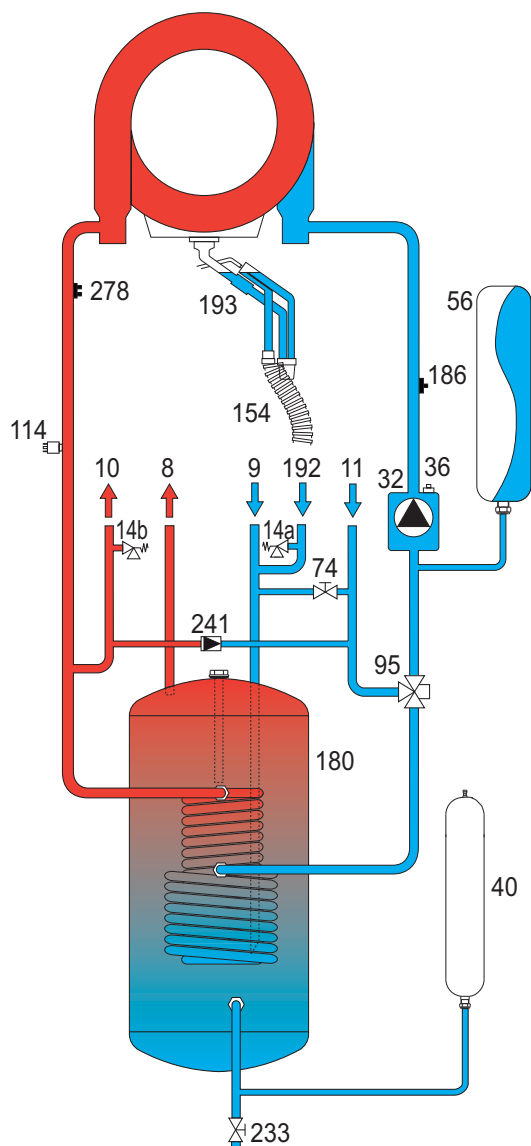
fig. 28 - Circuito idraulico
