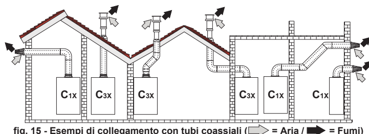
fig. 15 - Esempi di collegamento con tubi coassiali (→ = Aria / → = Fumi)
