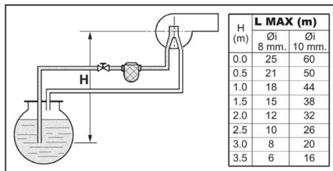
fig.19 - Alimentación por aspiración
