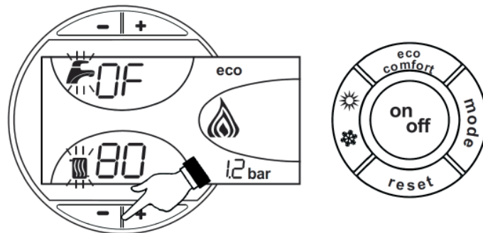
fig.24 - Modalità TEST
