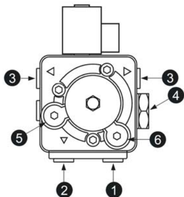
fig.25 - Pompa ITALPUMP
