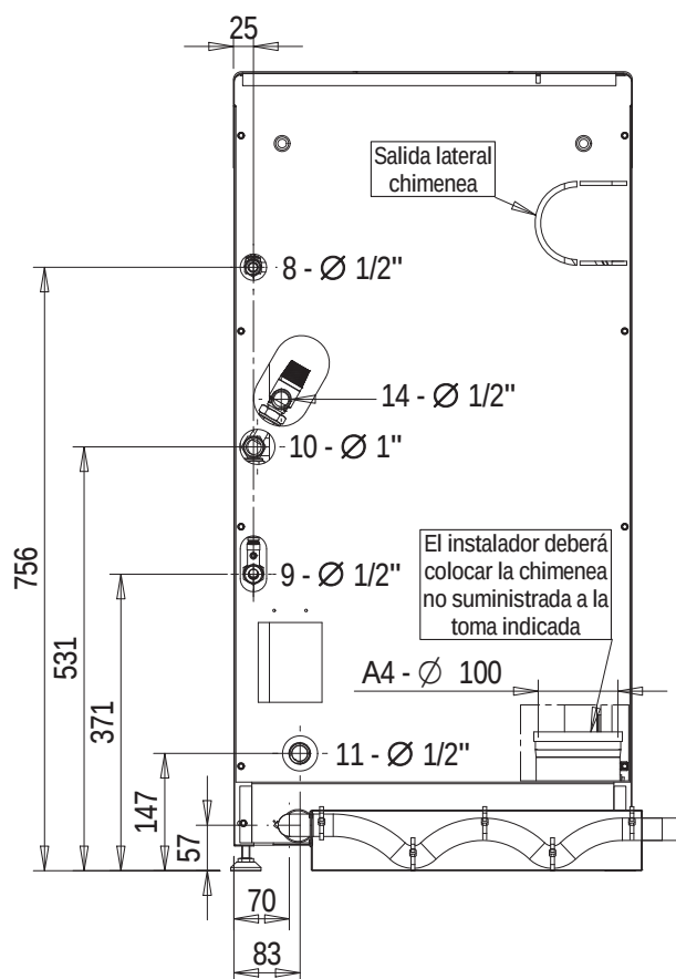
fig.38 - Vista posterior
