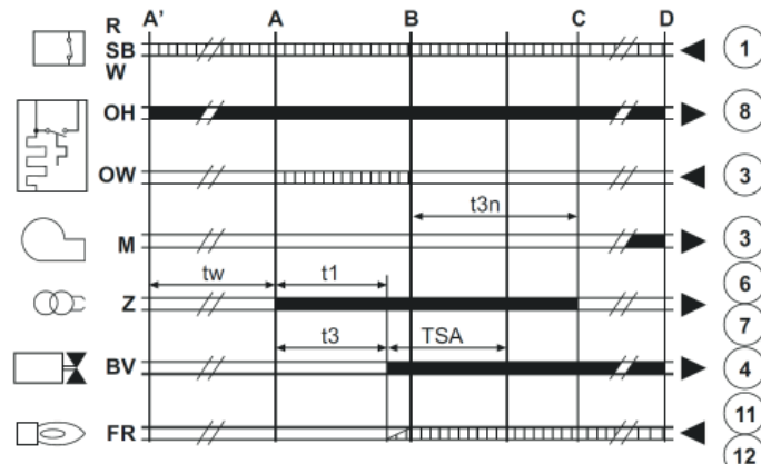
fig.31 - Ciclo dell'apparecchiatura
