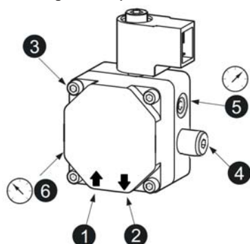
fig.26 - Pompa DANFOSS
