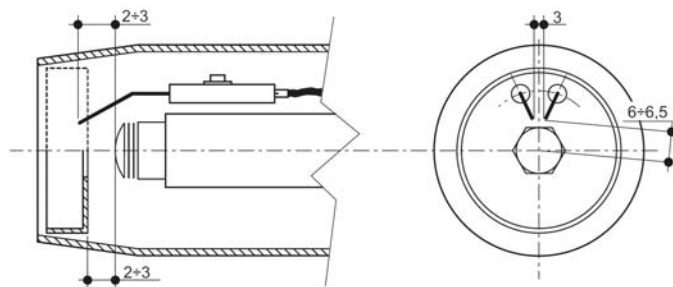
fig.29 - Posición de los electrodos y del deflector
