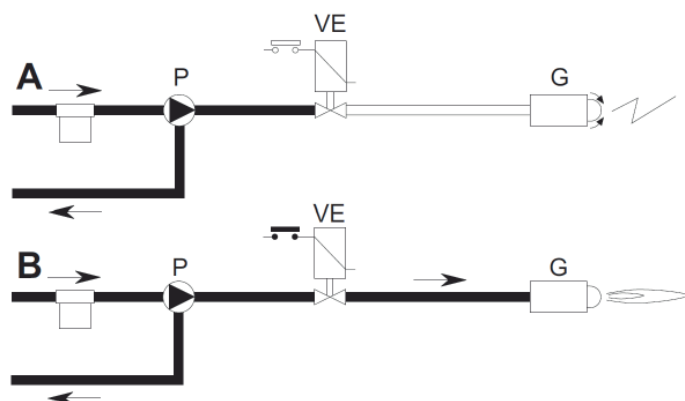
fig.30 - Encendido
