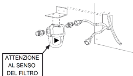
fig.18 – Installazione filtro combustibile
