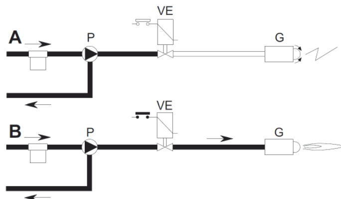
fig.30 - Avviamento
