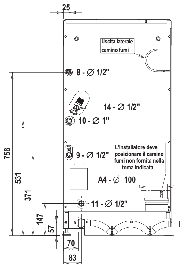
fig.38 - Vista posteriore
