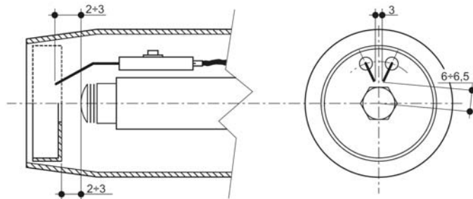
fig.29 - Posizione elettrodi - deflettore
