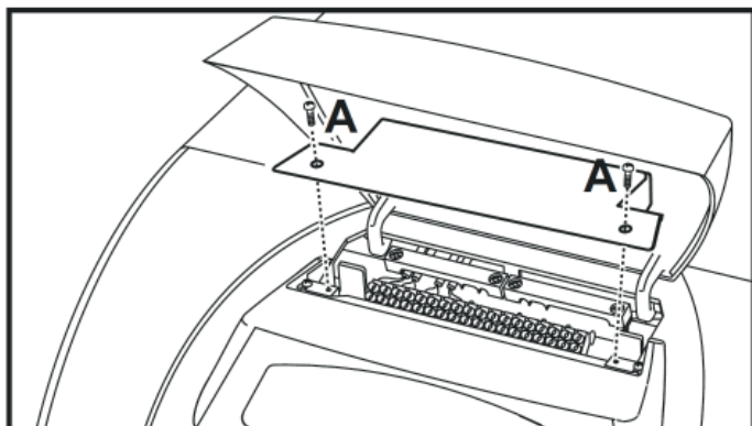
fig.22 - Acceso a la regleta de conexiones
