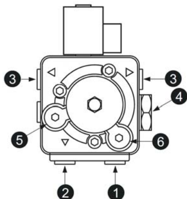
fig.25 - Bomba ITALPUMP
