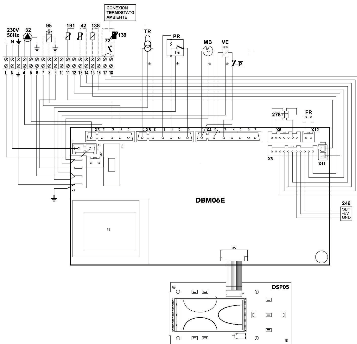
fig.42 - Esquema eléctrico
