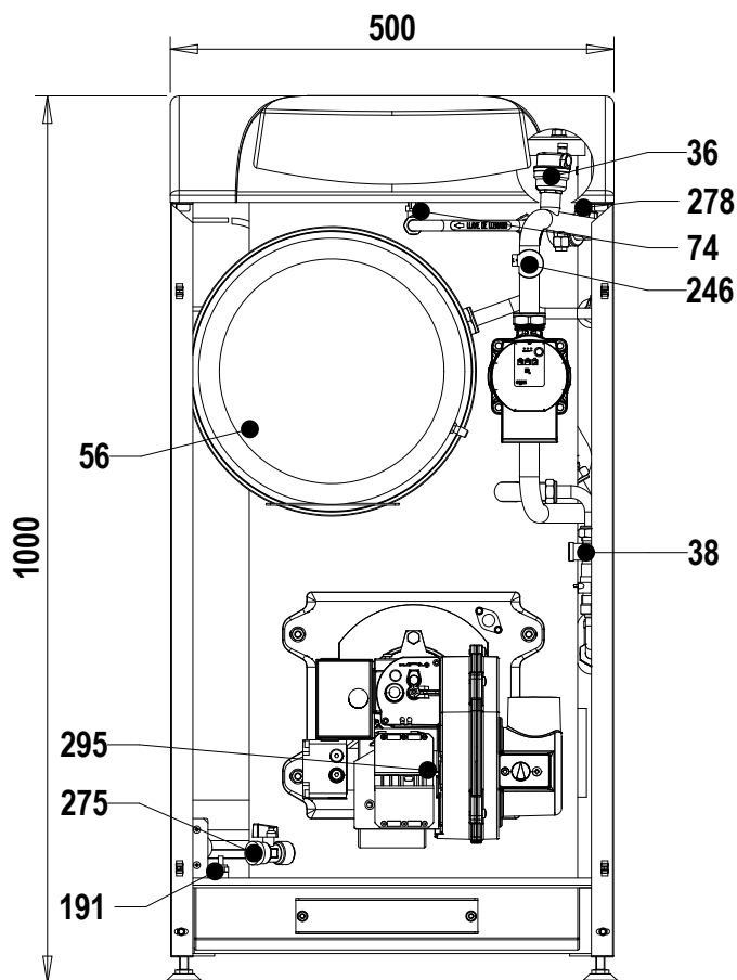
fig.37 - Vista frontale
