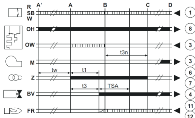
fig.31 - Ciclo del equipo
