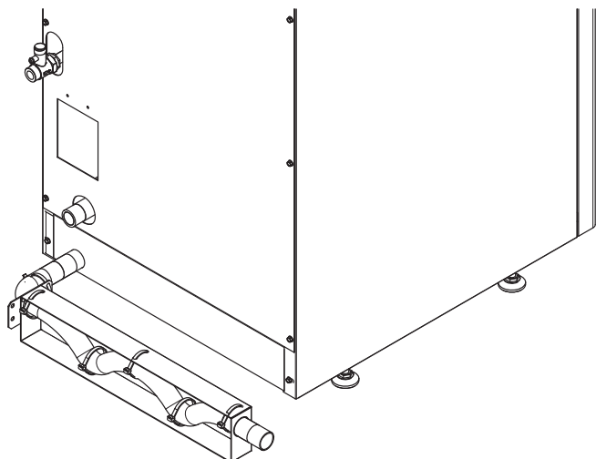
fig.23 - Condensate drain
