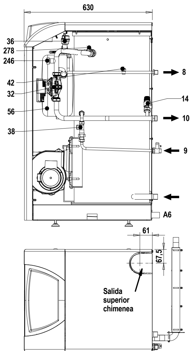
fig.36 - Vista lateral y superior
