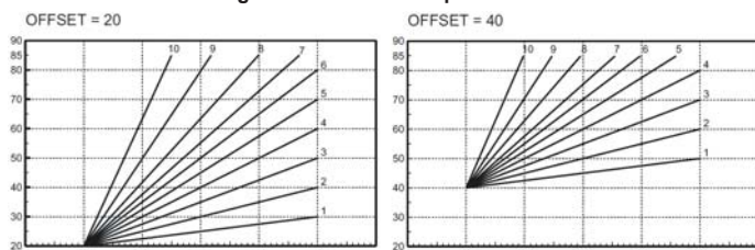
fig.15 - Ejemplo de desplazamiento paralelo de las curvas de compensación Ajustes del reloj programador a distancia
