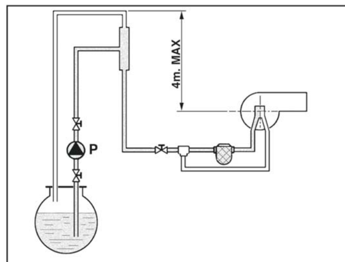
fig.21 - Alimentación en anillo
