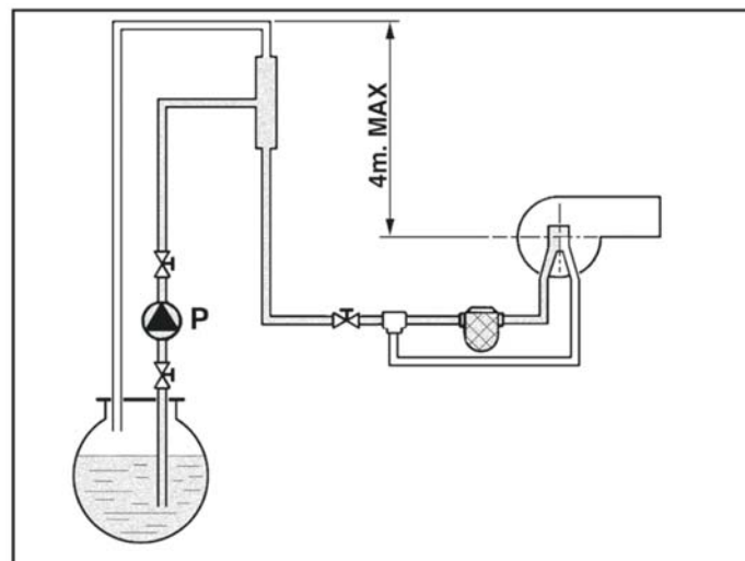
fig.21 – Alimentazione ad anello
