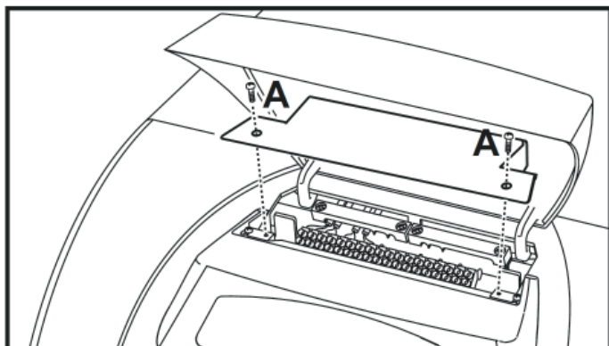
fig.22 – Accesso alla morsettiere
