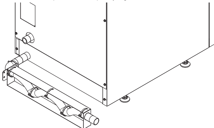
fig.23 - Descarga de condensados
