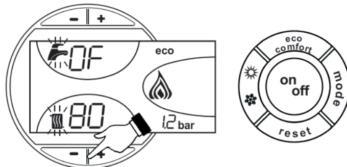
fig.24 - Modo TEST
