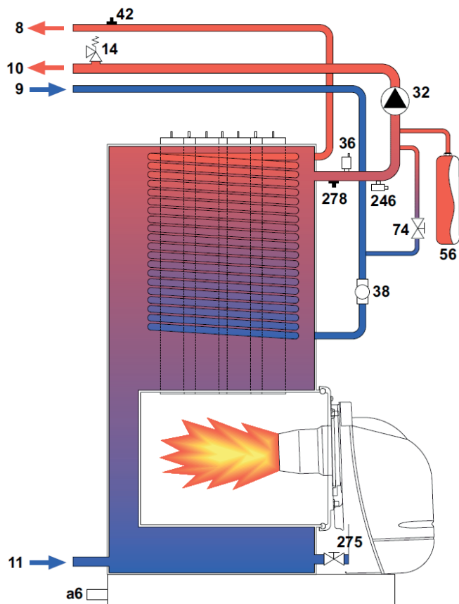
fig.39 - Circuito idraulico
