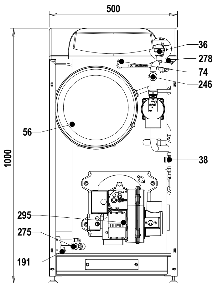
fig.37 - Vista frontal
