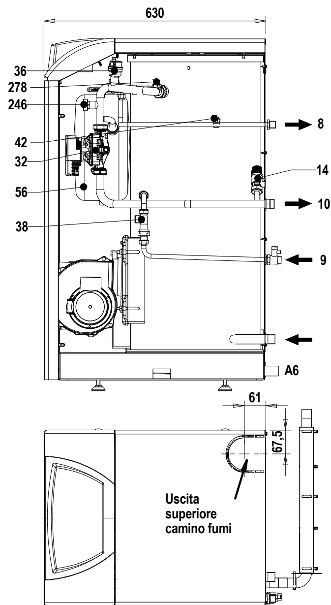
fig.36 - Vista laterale e superiore
