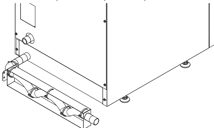
fig.23 - Scarico condensa
