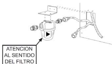
fig.18 - Instalación del filtro del combustible
