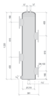
Collettori collegamento idraulico separatore DN 100 042088X0
