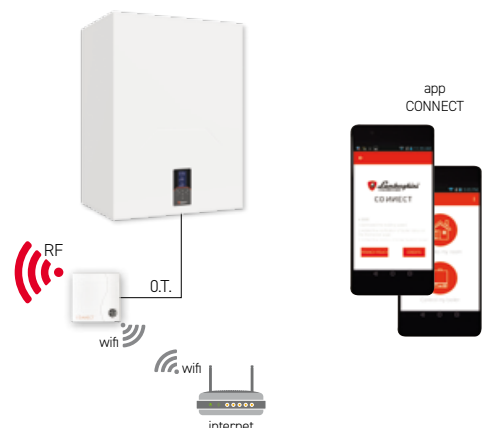
Ricevitore RF/WiFi
