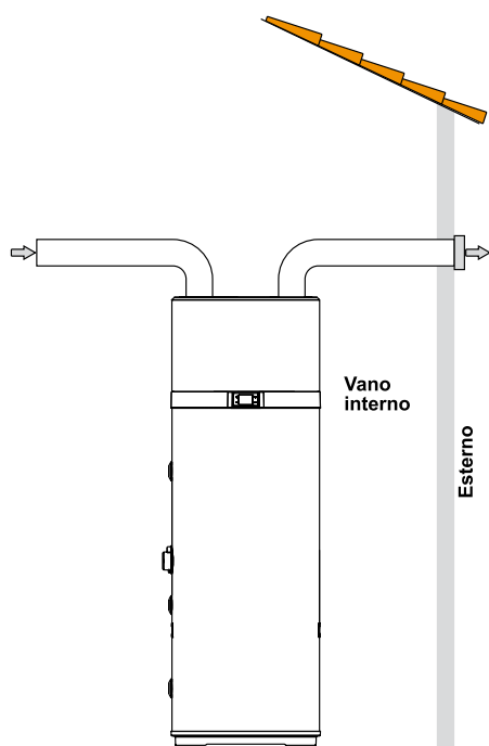
Fig. 1 Esempio di collegamento scarico aria (questo tipo di installazione può essere realizzato solo con mod. 200 e 260)
