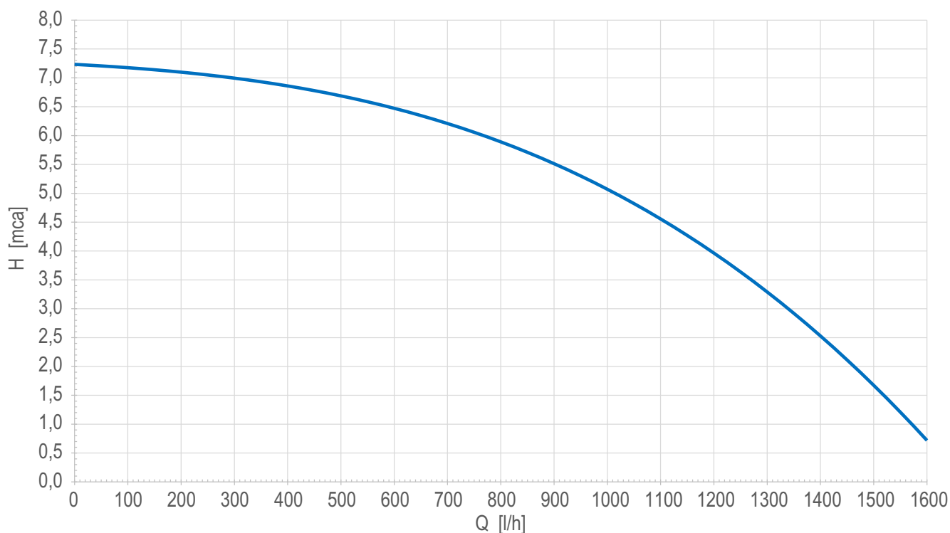
slika 59- Preostala potisna visina raspoloživa u instalaciji
