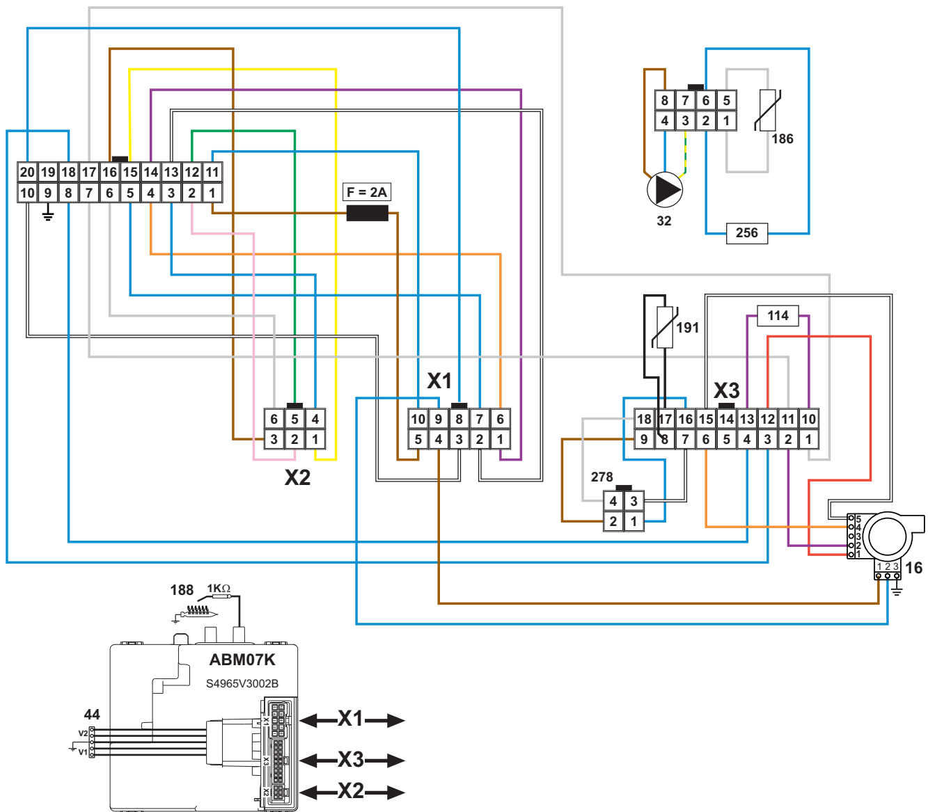
fig. 120 - Schema elettrico Primo modulo
