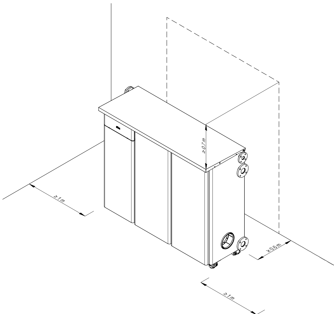
fig. 37 - Posizionamento con distanze da rispettare
