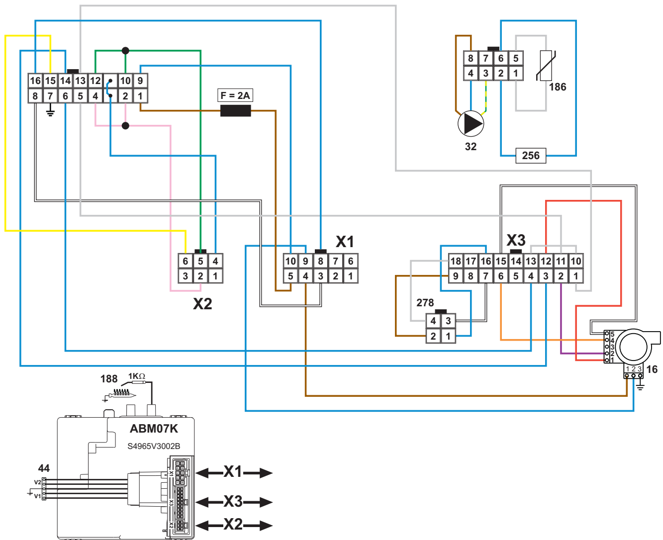
fig. 122 - Schema elettrico Ultimo modulo
