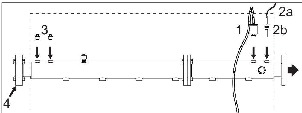
fig. 41 - Mandata a destra
