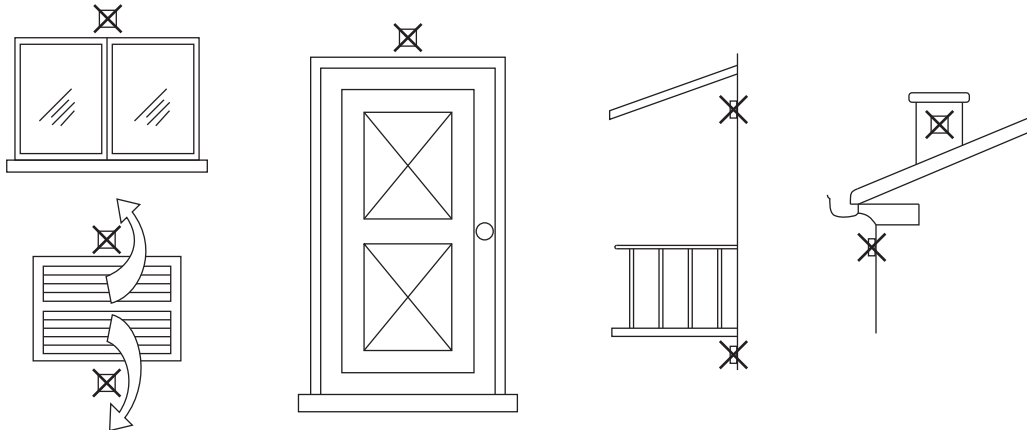
fig. 68 - Posizionamento sconsigliato sonda esterna
