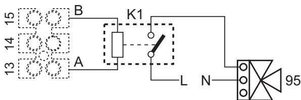
fig. 116 - Collegamento della valvola a 3 vie con 2 fili
