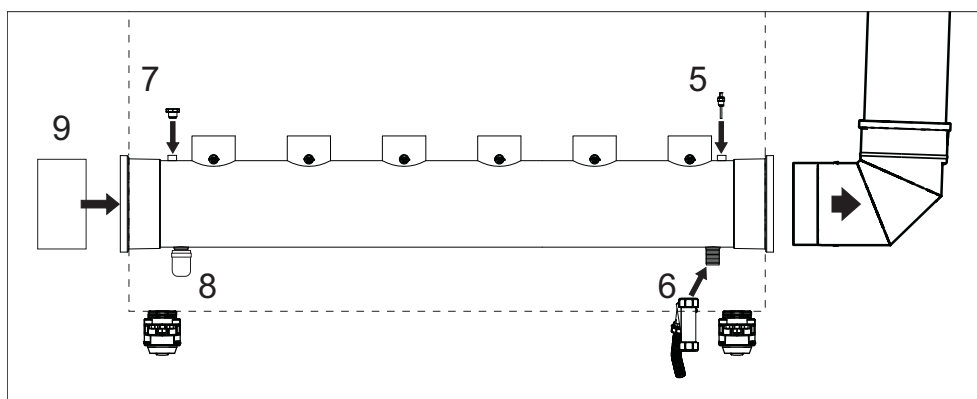
fig. 44- Right side fumes outlet
