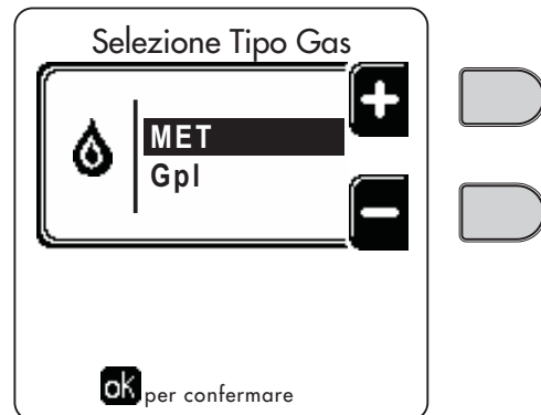
fig. 85 - Selezione tipo di gas
