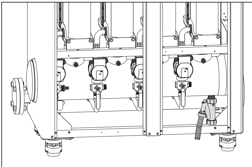
fig. 76 - Collegamento scarico condensa
