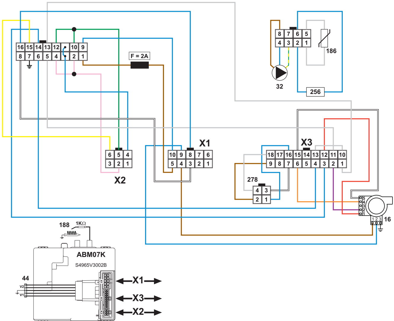
fig. 122- Last module wiring diagram
