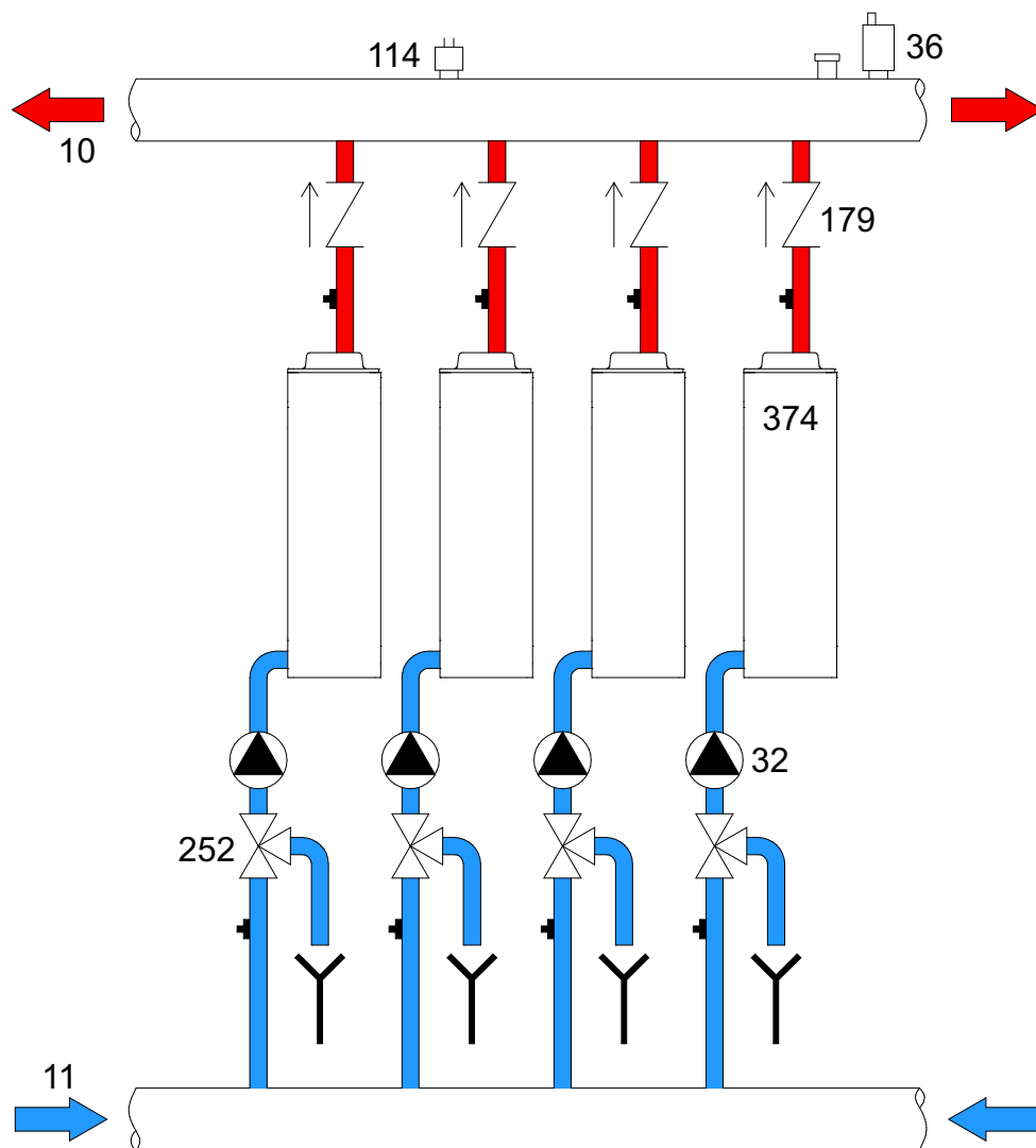
fig. 115 - Circuito idraulico
