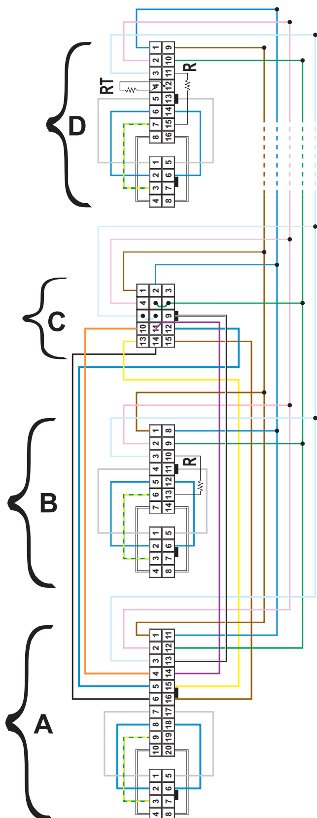
fig. 123 - Schema elettrico Cavo di collegamento moduli
