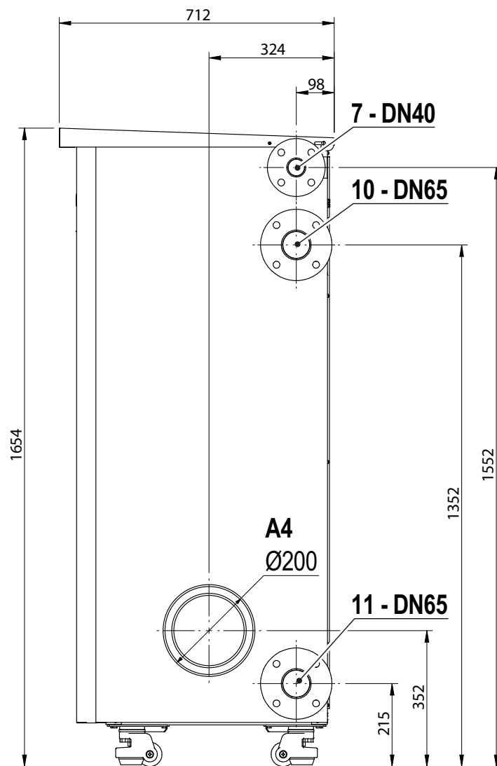
fig. 113 - Vista laterale
