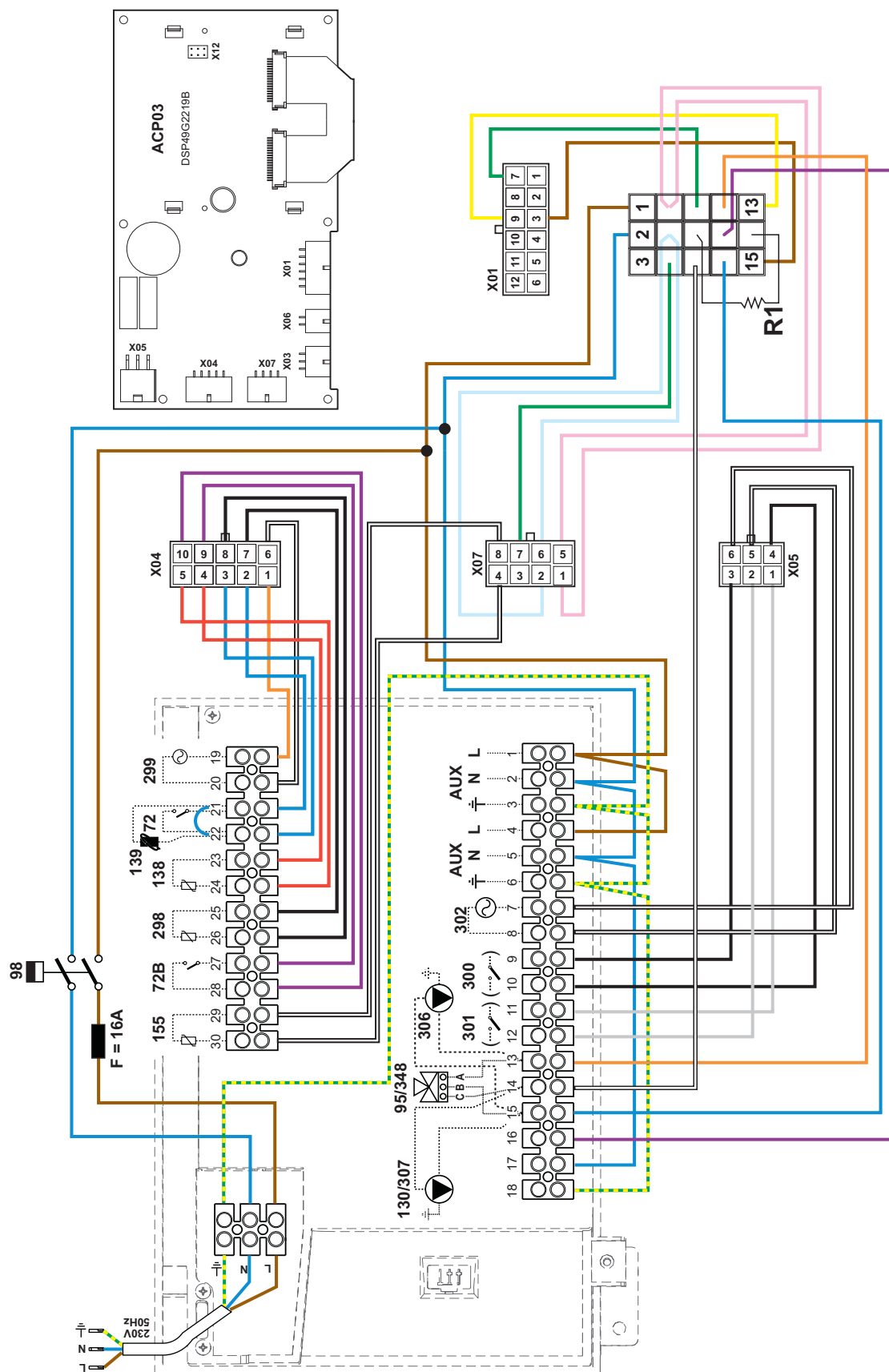
fig. 119 - Schema elettrico Display
