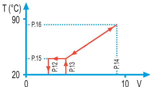
fig. 51 - Controllo in temperatura
