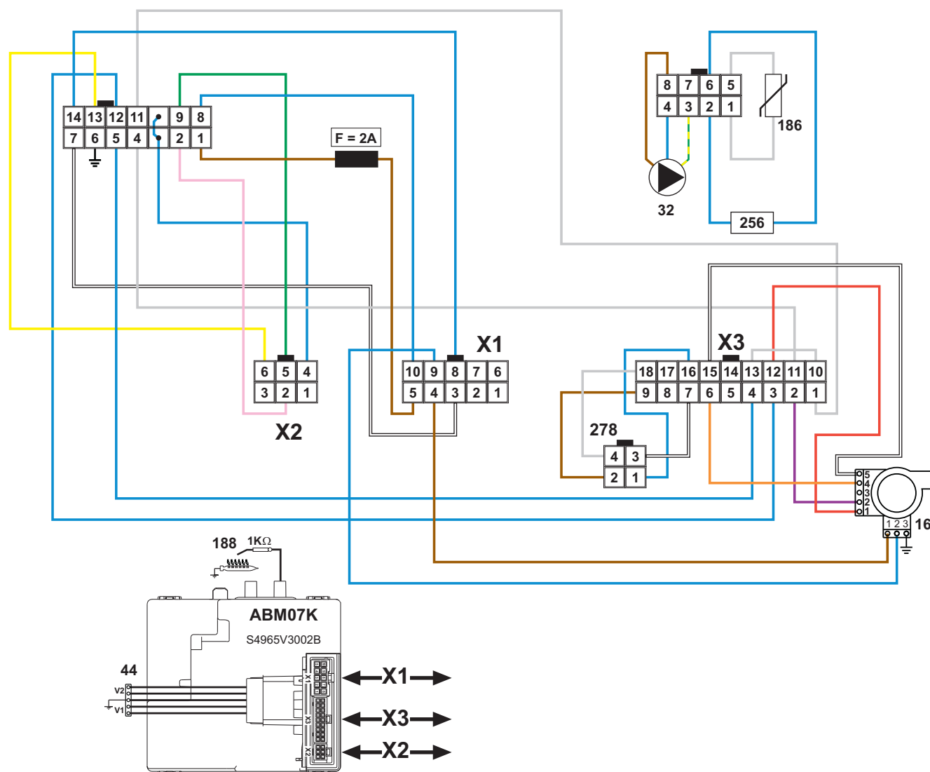
fig. 121 - Schema elettrico Modulo intermedio
