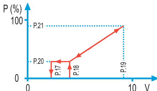
fig. 52 - Controllo in potenza
