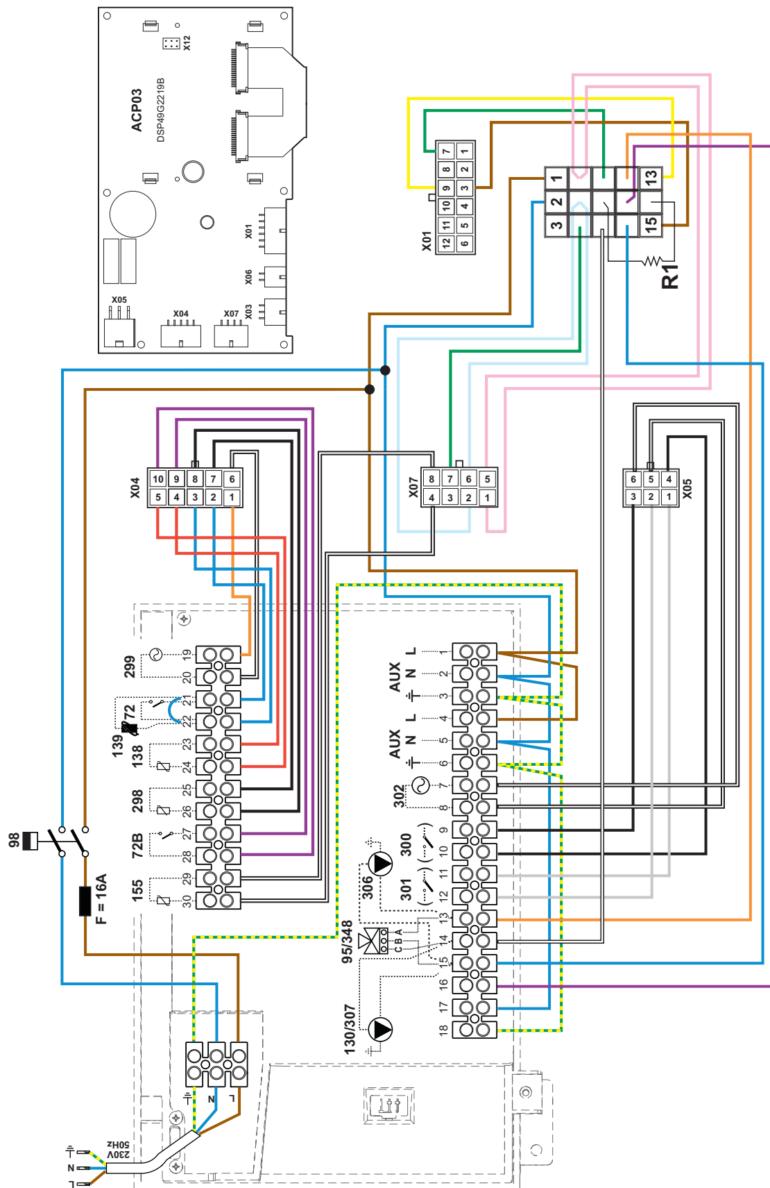
fig. 119- Display wiring diagram
