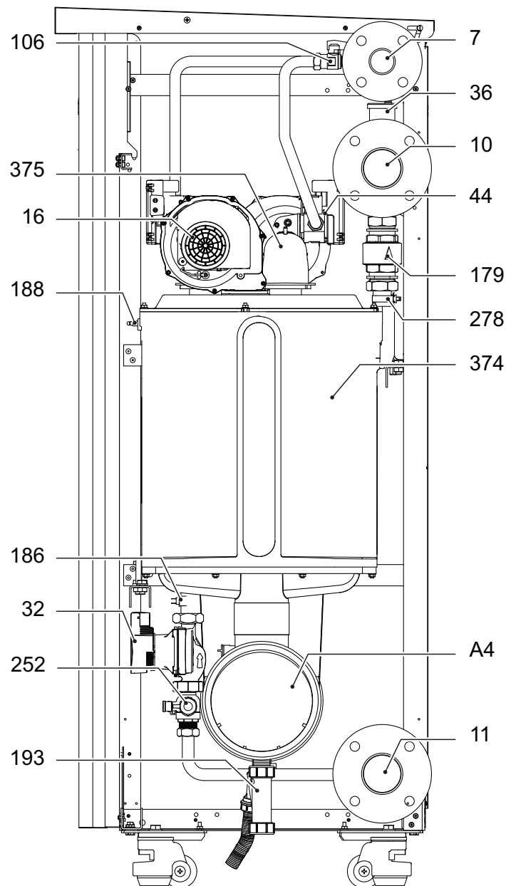
fig. 114 - Componenti principali
