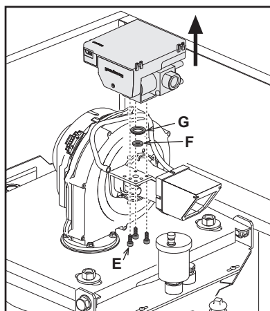
fig. 59 - Modello CLOVER 70
