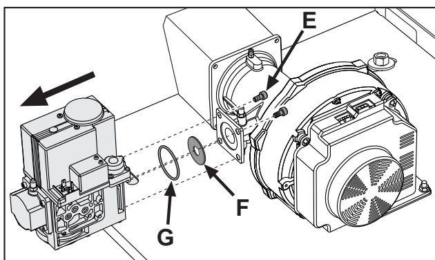
fig. 62- Modelo CLOVER 320
