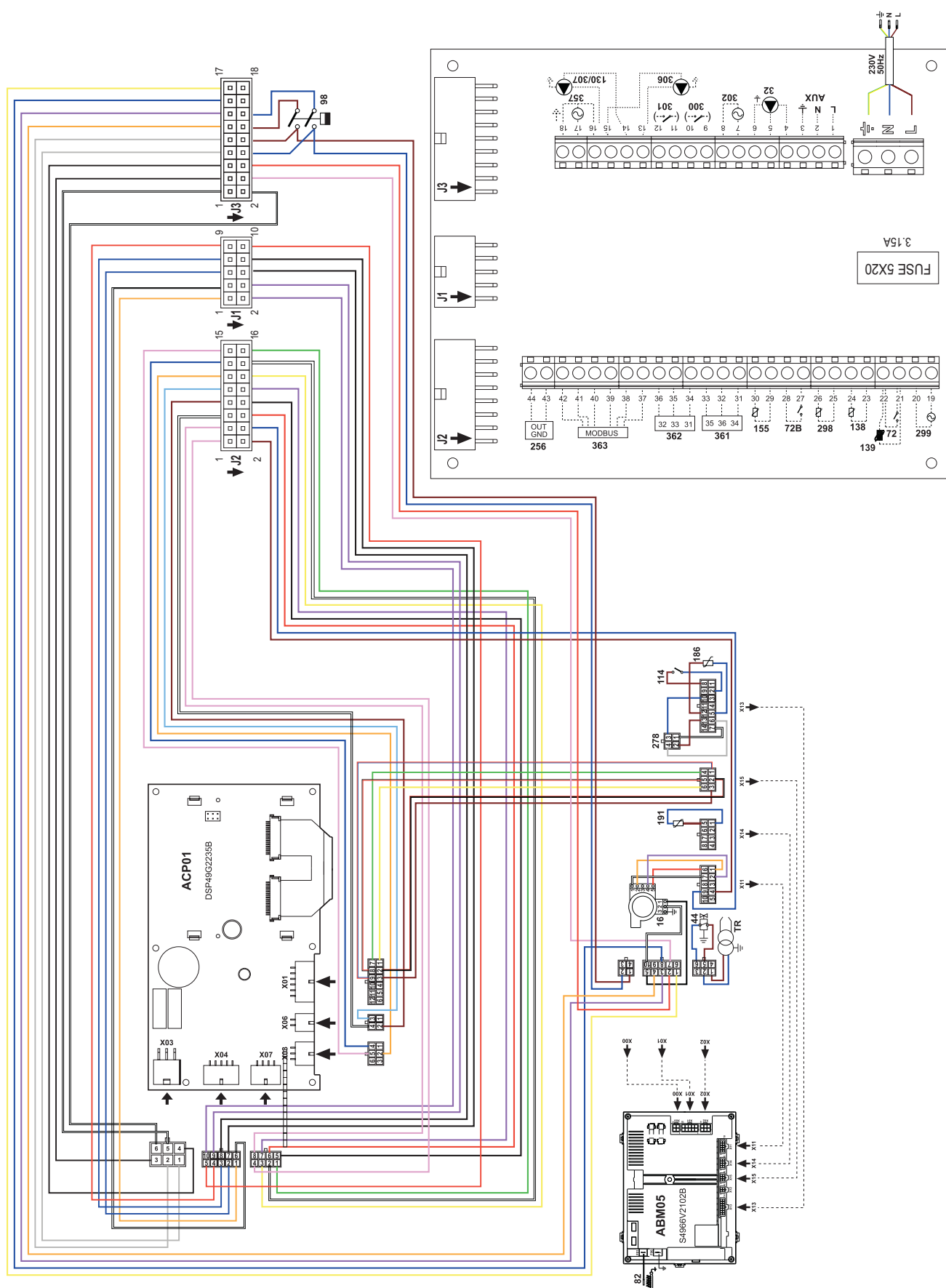
fig. 94 - Schema elettrico CLOVER 220/320
