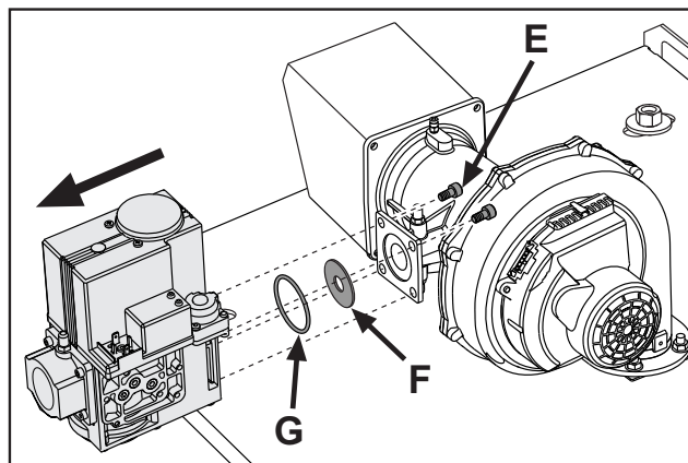
fig. 61- Modelo CLOVER 220
