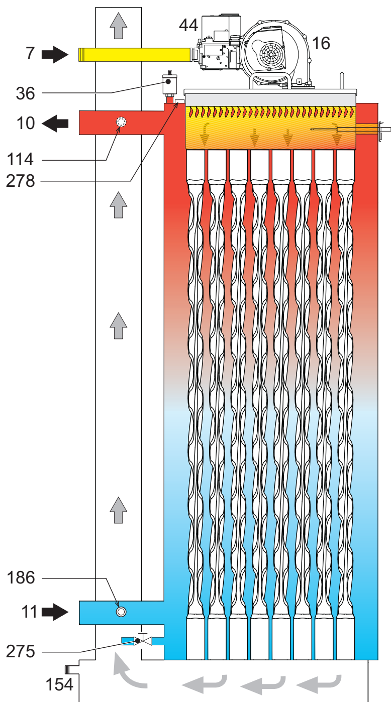
fig. 86- Circuito hidráulico
