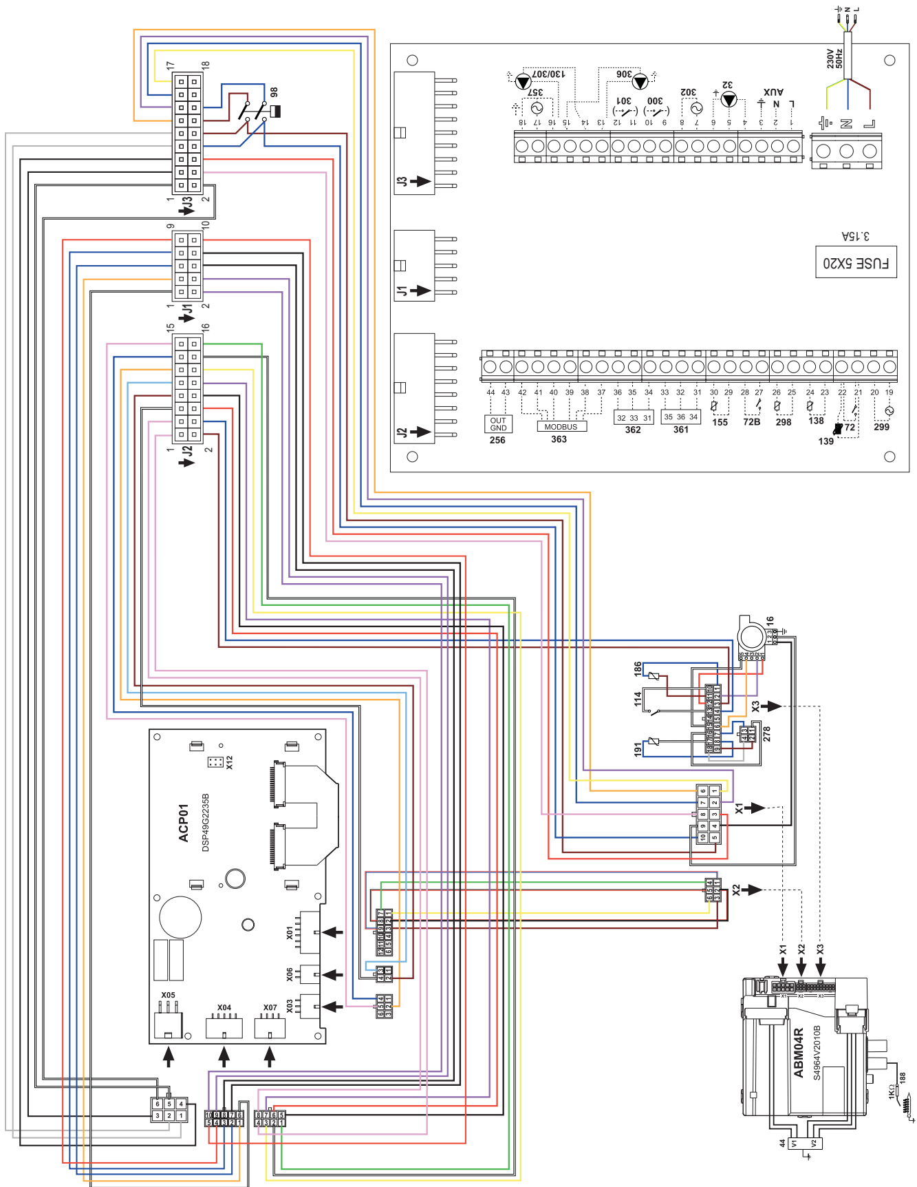
fig. 93- Schéma électrique CLOVER 125 et 160
