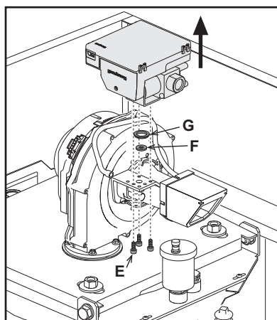
fig. 59- Modelo CLOVER 70
