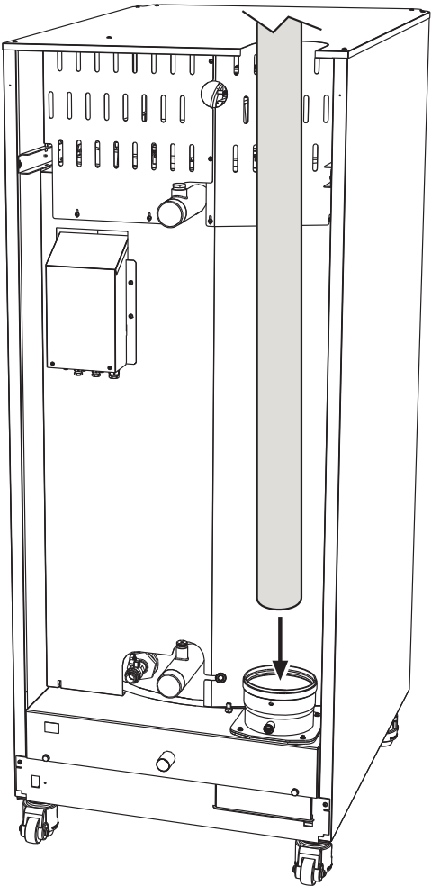
fig. 57- Fume outlet
