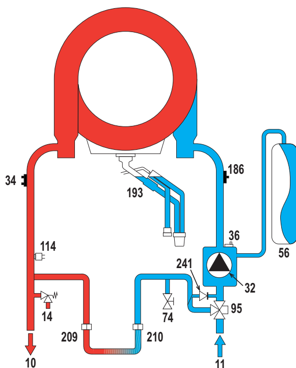
fig. 56 - Circuito idraulico
