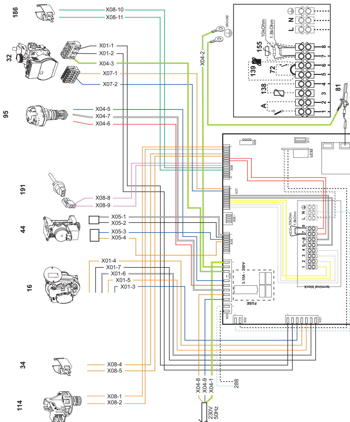
fig. 58 - Schema elettrico
