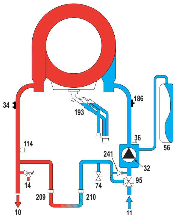
рис. 56- Гидравлический контур
